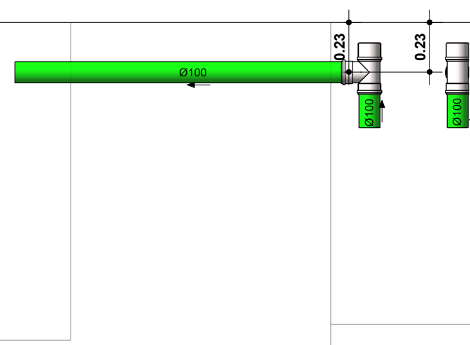
DETALHE - TANQUE SÉPTICO E SUMIDOURO
