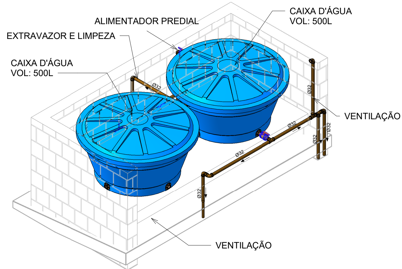
1 DETALHE-CAIXA D'ÁGUA
