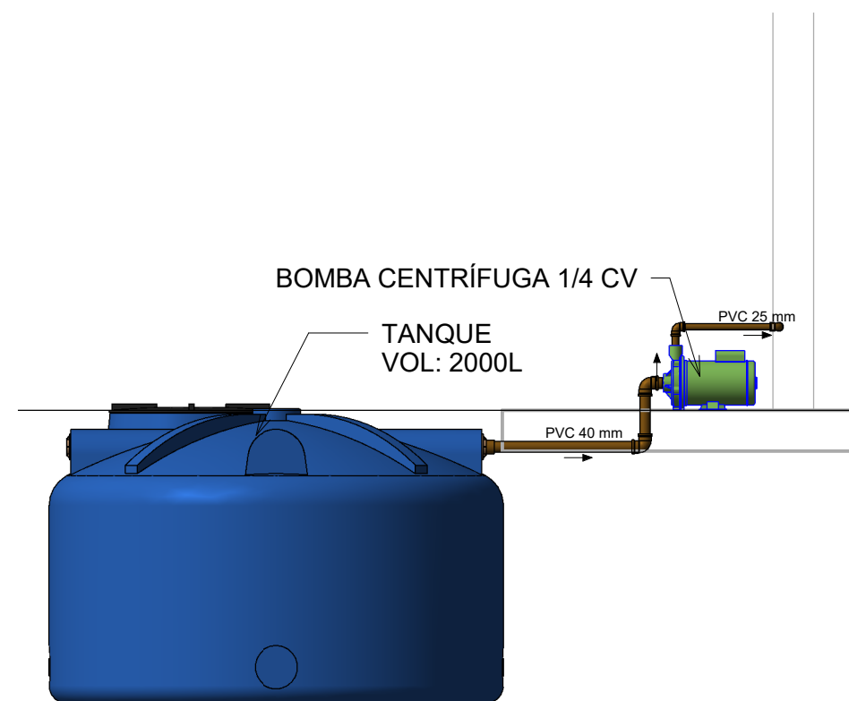
DETALHE - CASA DE BOMBA 1 : 25
