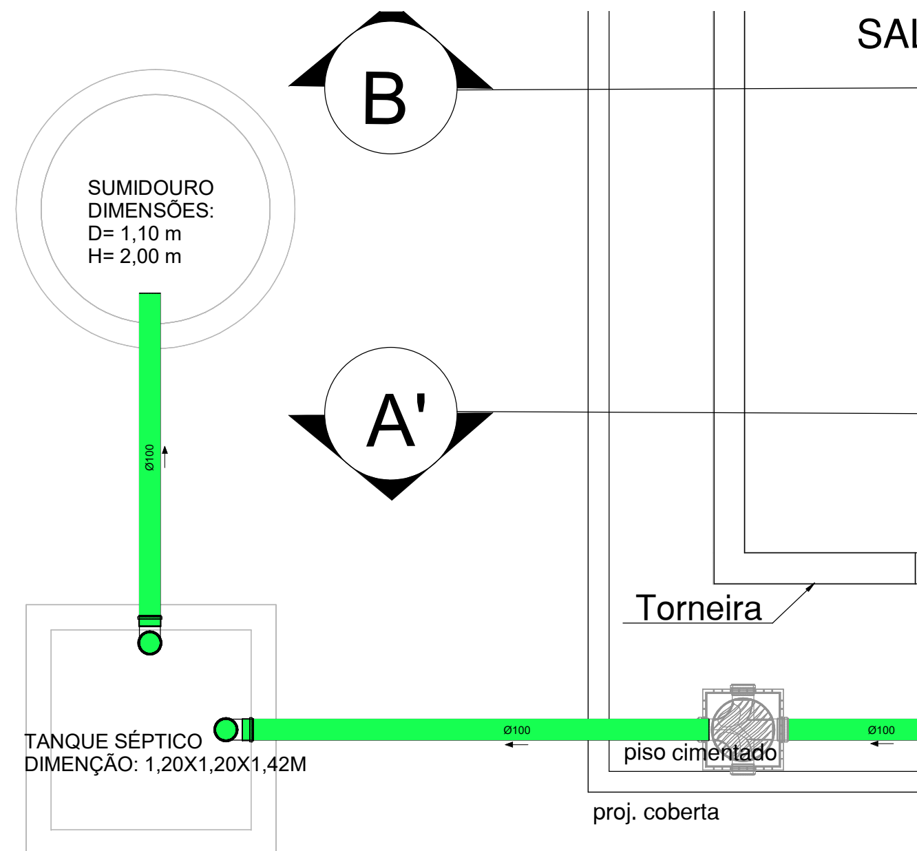
NÍVEL TÉRREO - ESGOTO - SUMIDOURO
