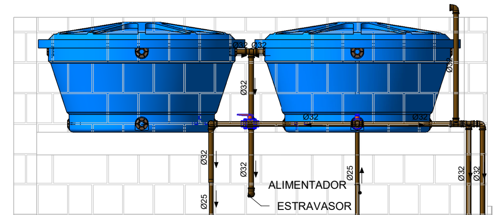
2 DETALHE-CAIXA D'ÁGUA
