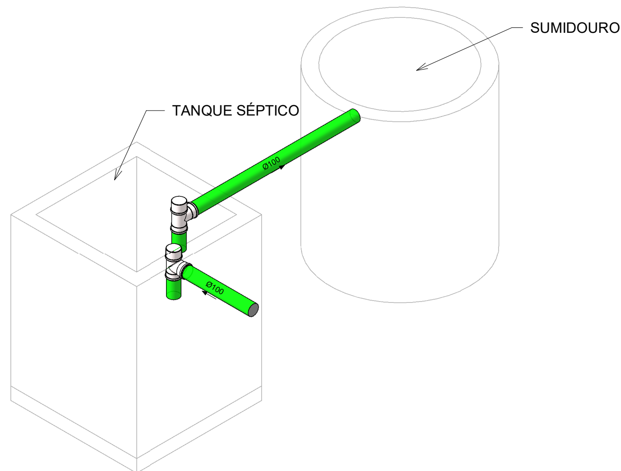
DETALHE - TANQUE SÉPTICO E SUMIDOURO
