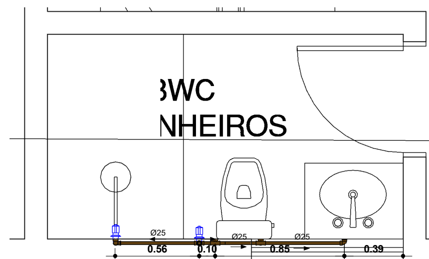
3 PLANTA BAIXA - ÁGUA FRIA 1 : 25
