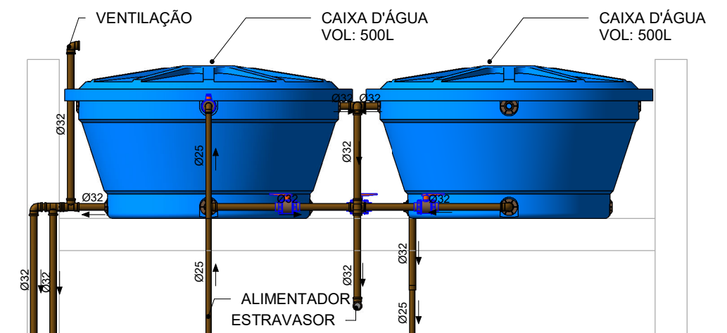
3 DETALHE - CAIXA D'ÁGUA
