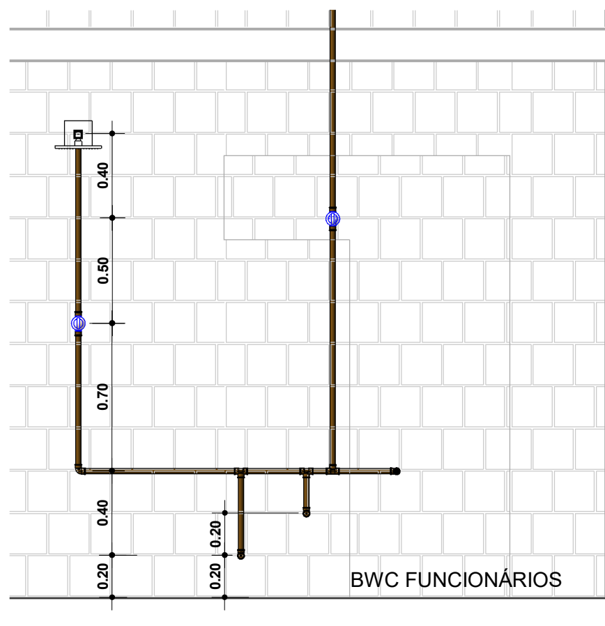
1 DETALHE 01 1 : 25
