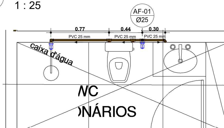
3 BWC FUNCIONÁRIOS 1 : 25
