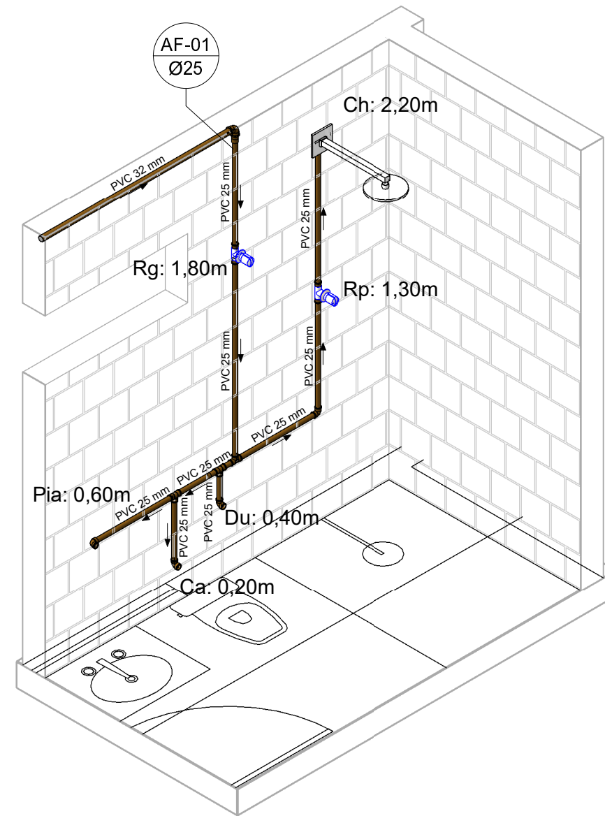
2 ISOMÉTRICO-BWC-ENGENHEIROS
