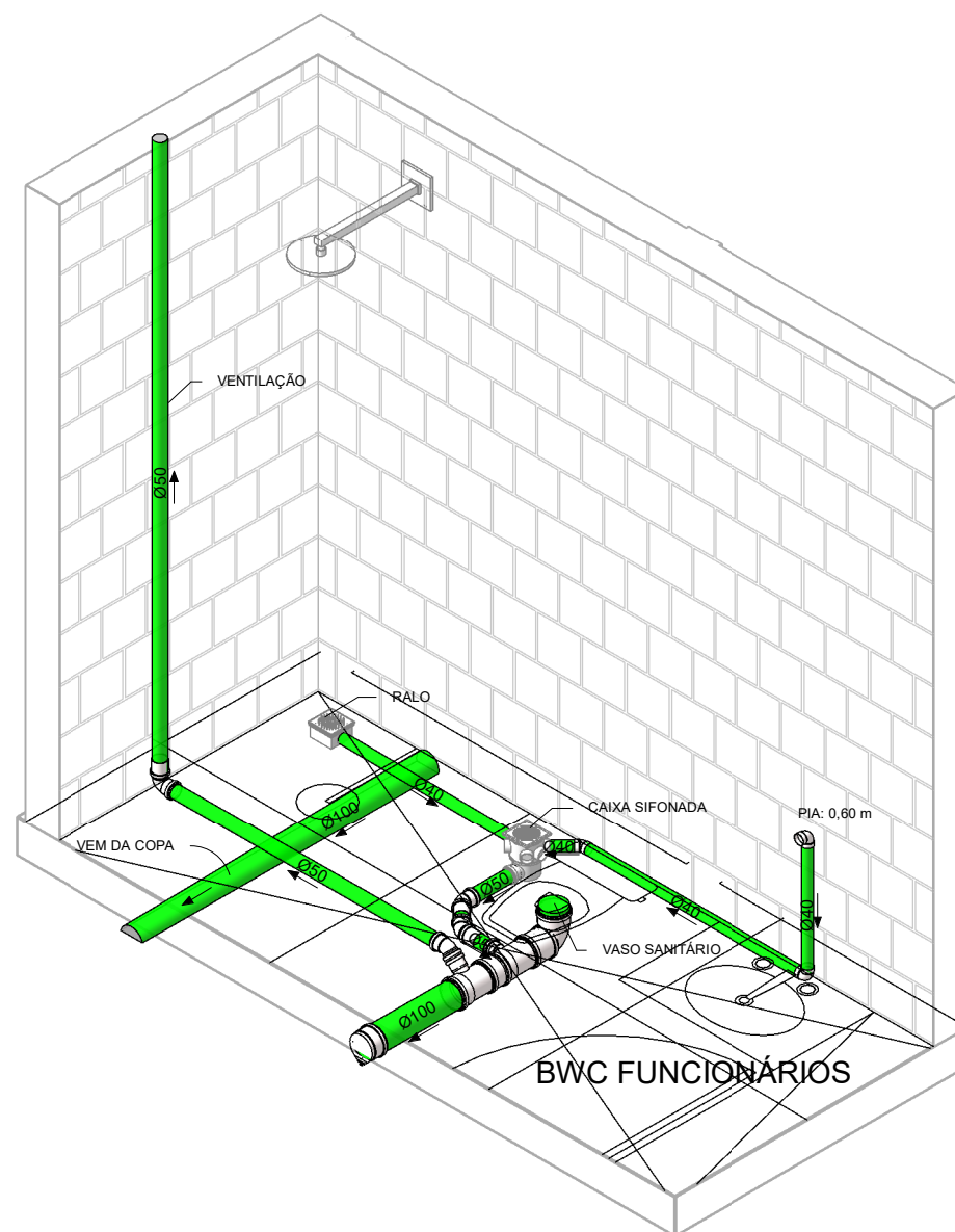
2 ISOMÉTRICO - ESGOTO - BWC - FUNCIONÁRIOS
