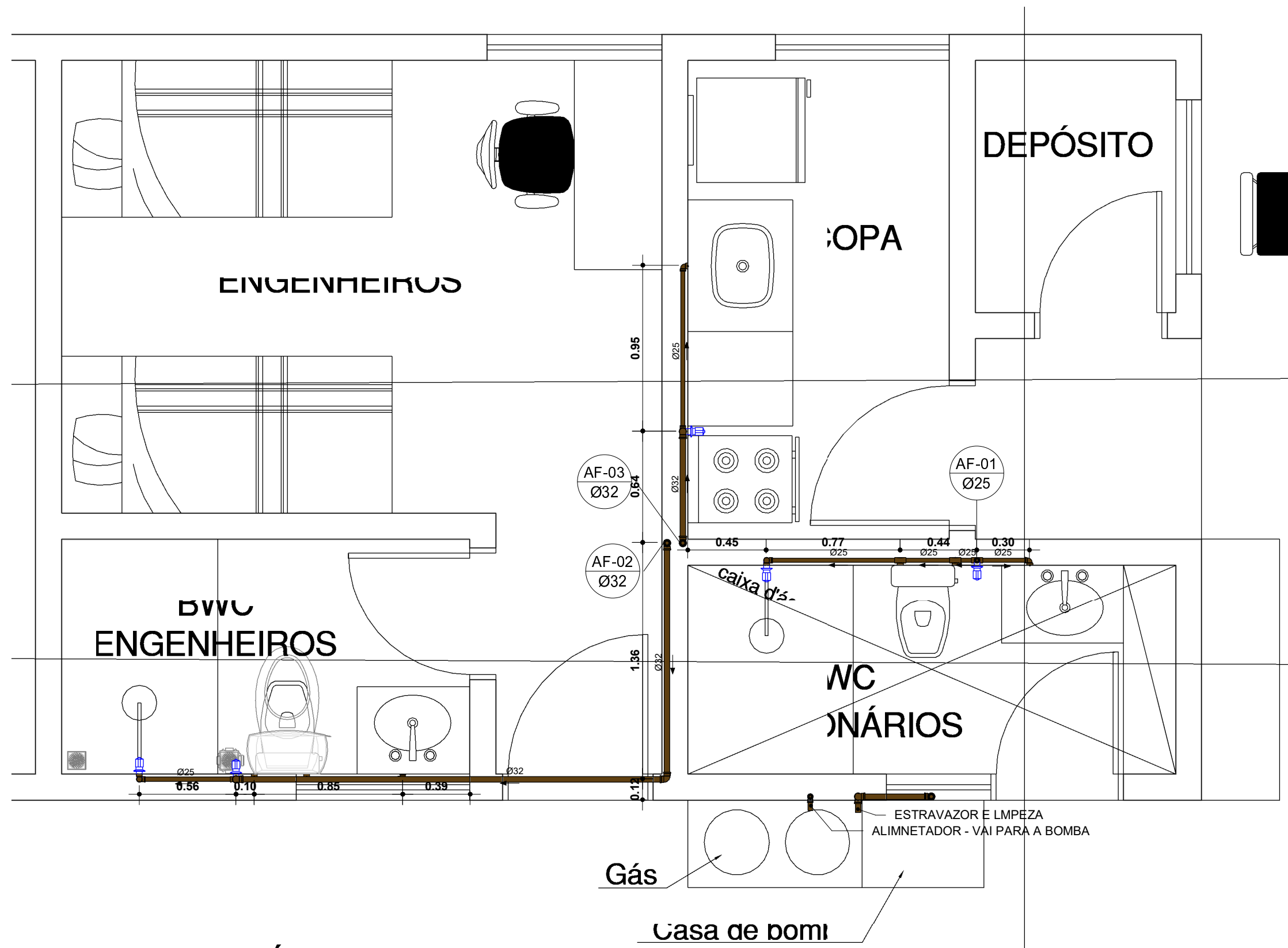
1 Nível Térreo - Água fria 1 : 25
