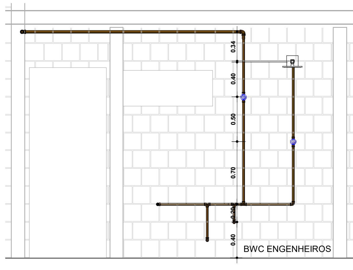
1 DETALHE 02 1 : 25
