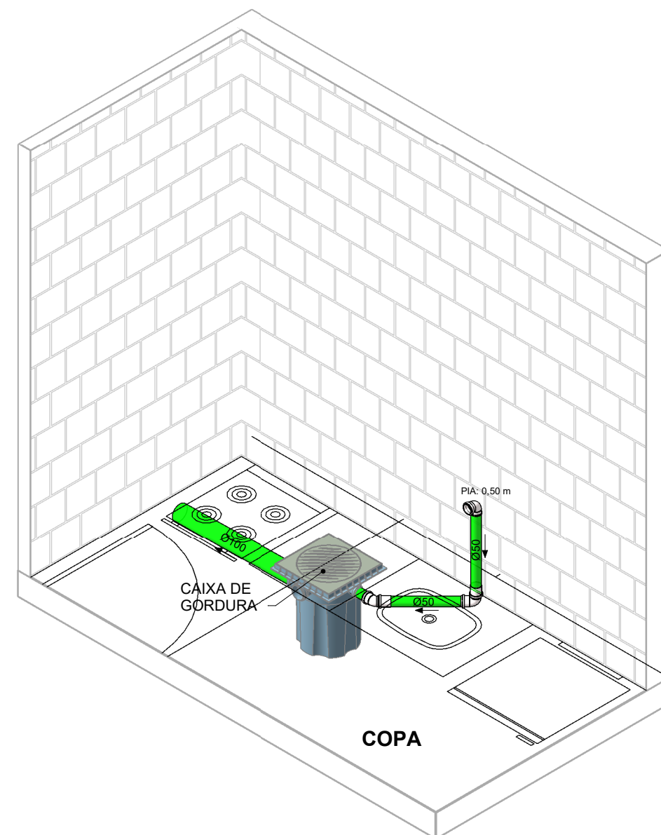
3 ISOMÉTRICO - ESGOTO - COPA
