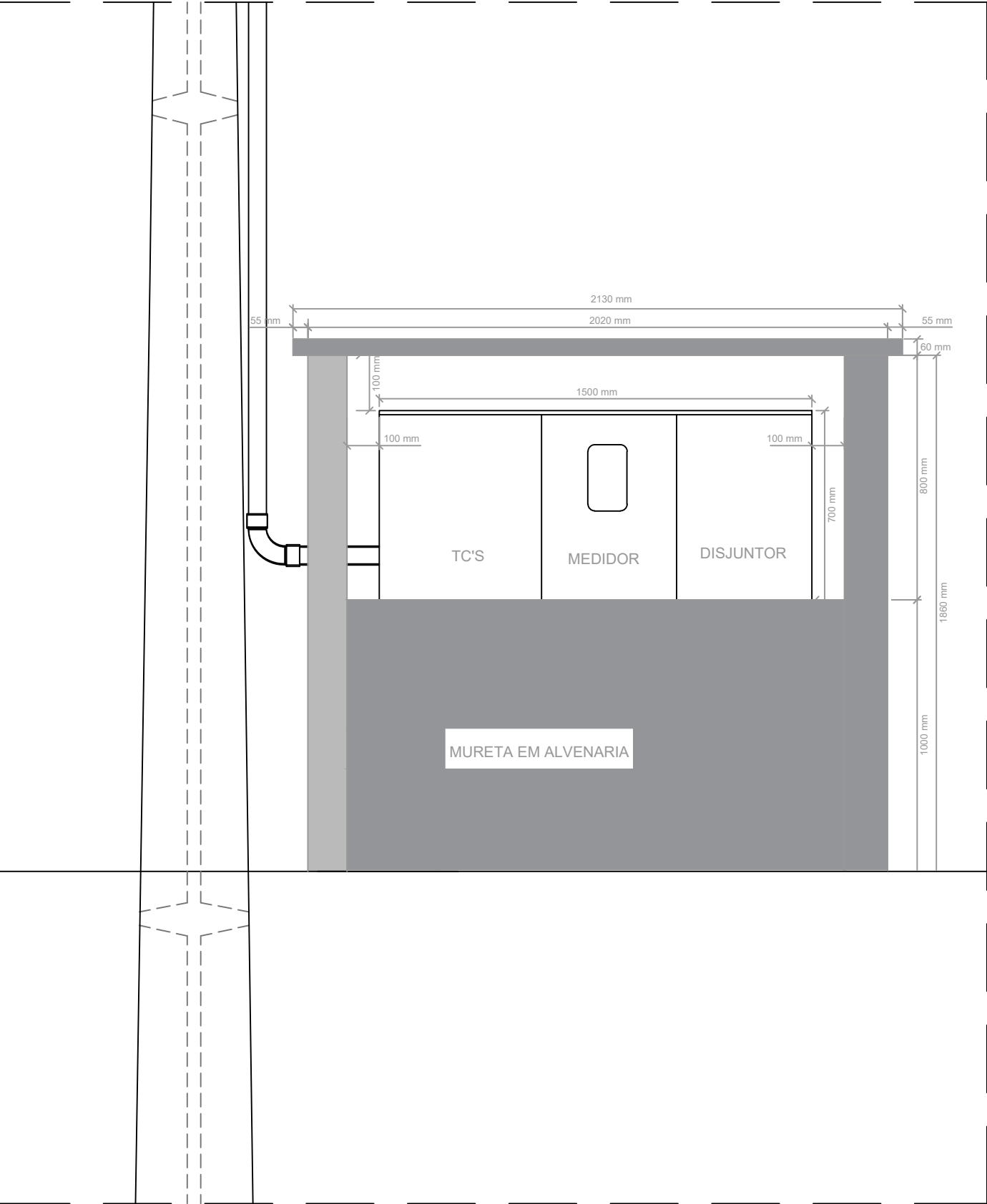
03 DETALHE DA MURETA DE MEDIÇÃO ESC.: 1/20
