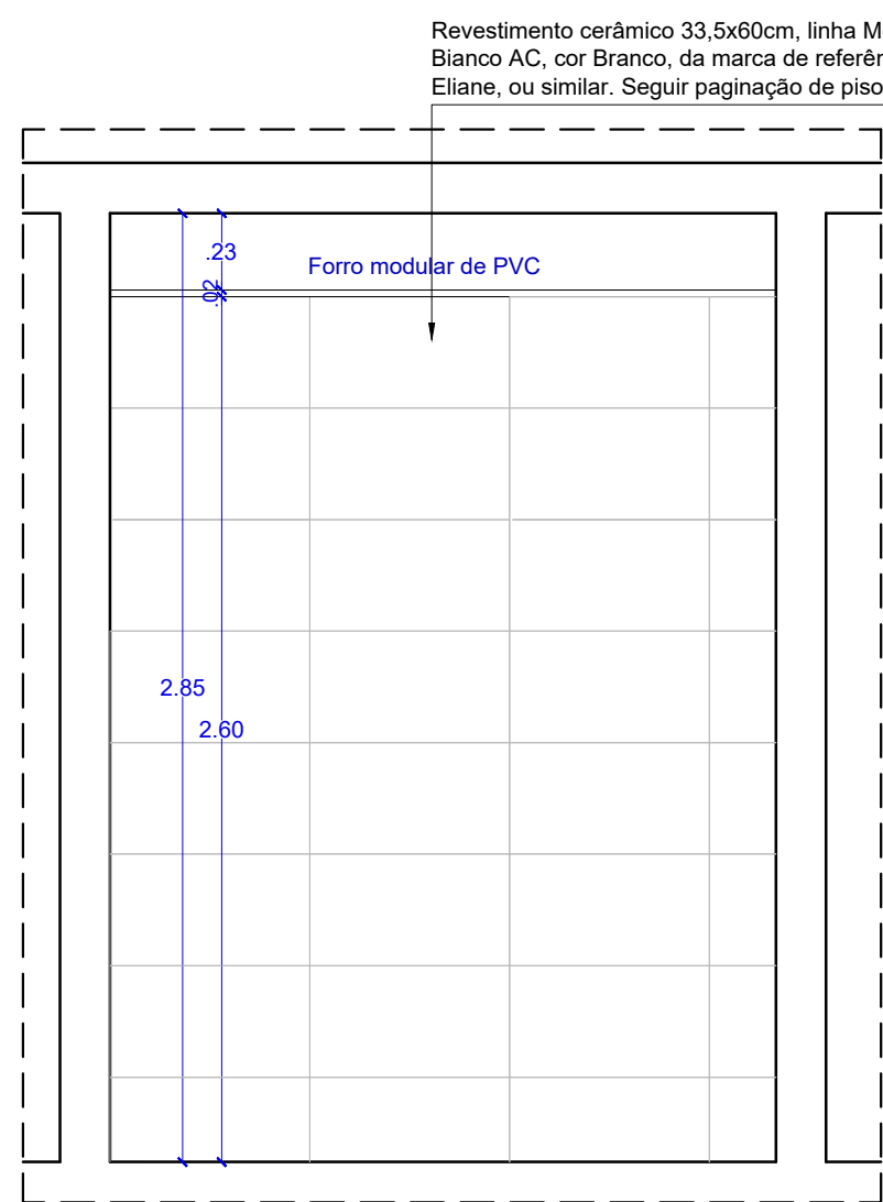
VISTA 02 WC PCD 1  PAV. ESCALA.....1/25
