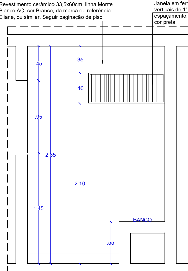
VISTA 03 CELTA ESCALA.....1/25
