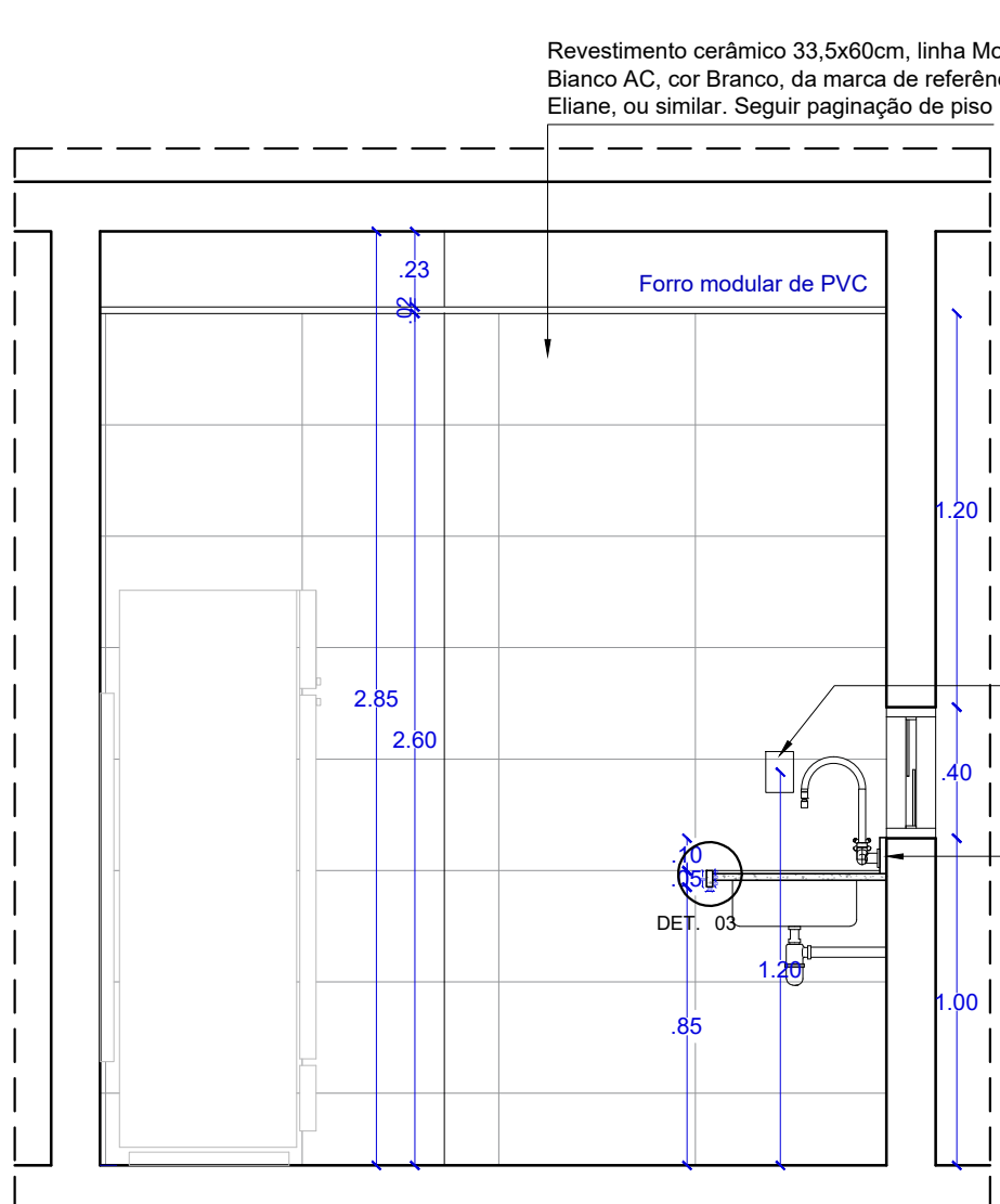
VISTA 03 COPA 1º PAV. ESCALA.....1/25
