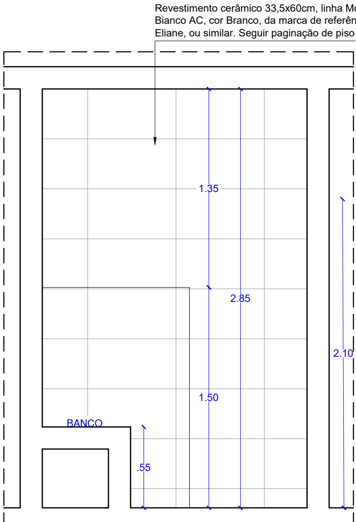
VISTA 01 CELTA ESCALA.....1/25
