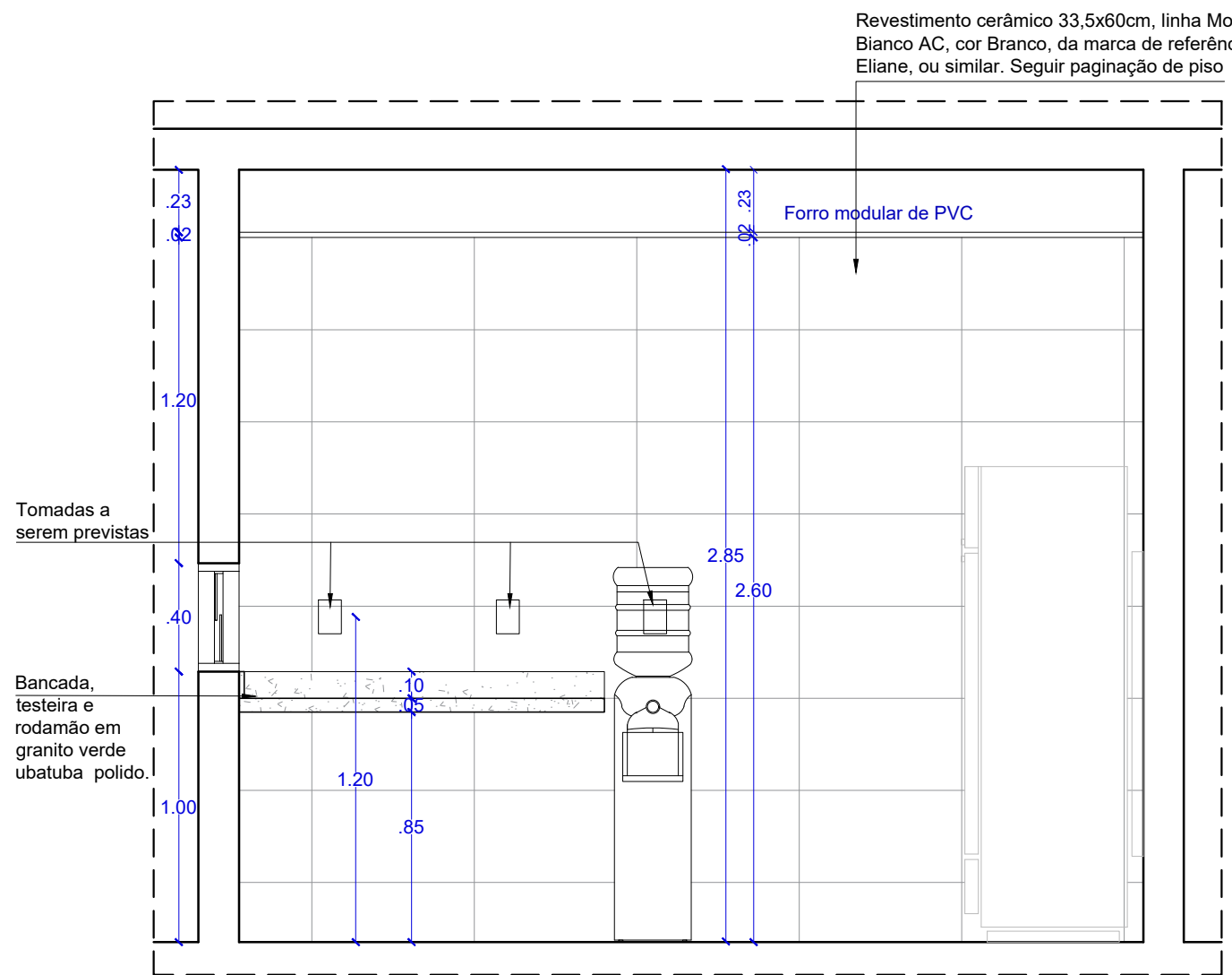
VISTA 01 COPA TÉRREO ESCALA.....1/25
