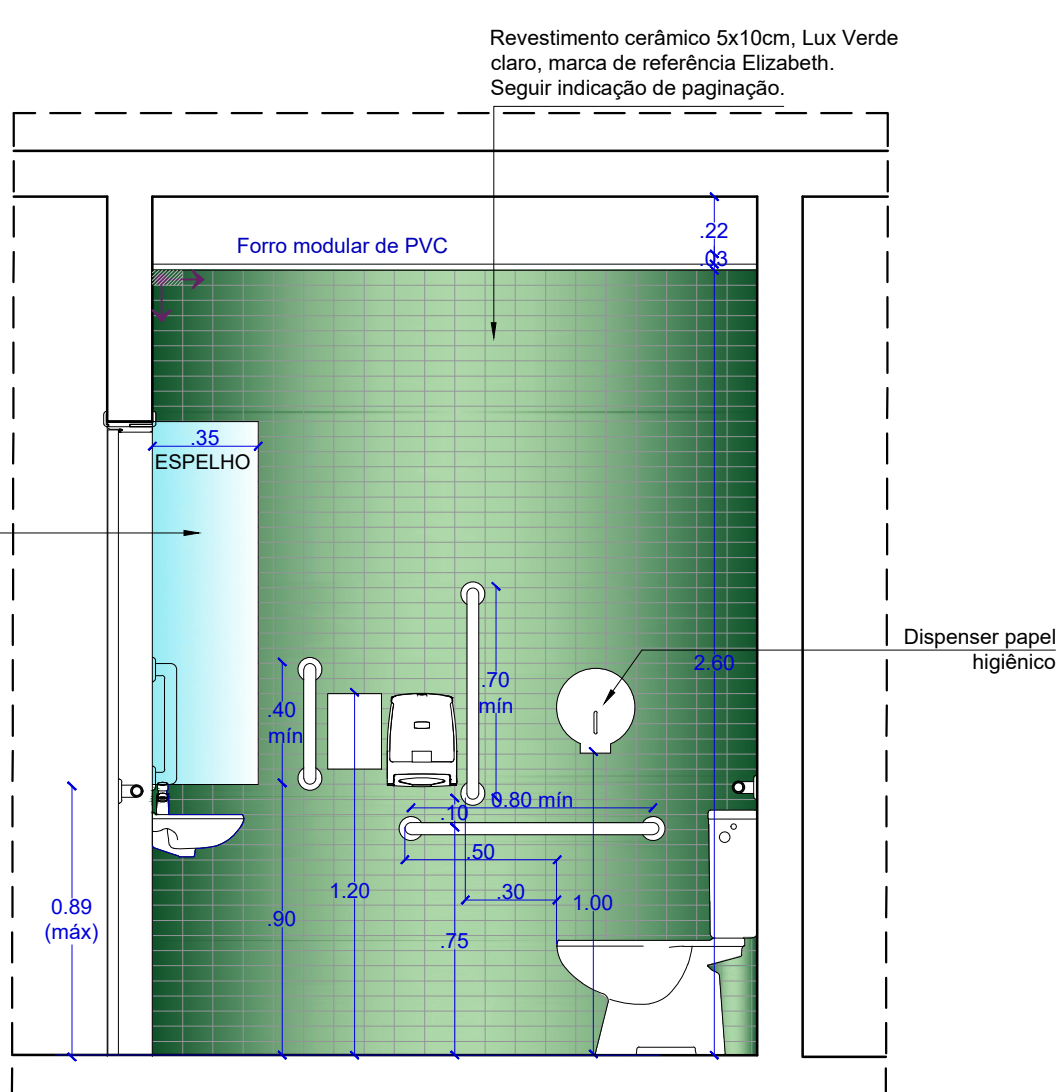
VISTA 04 WC PCD T RREO ESCALA.....1/25
