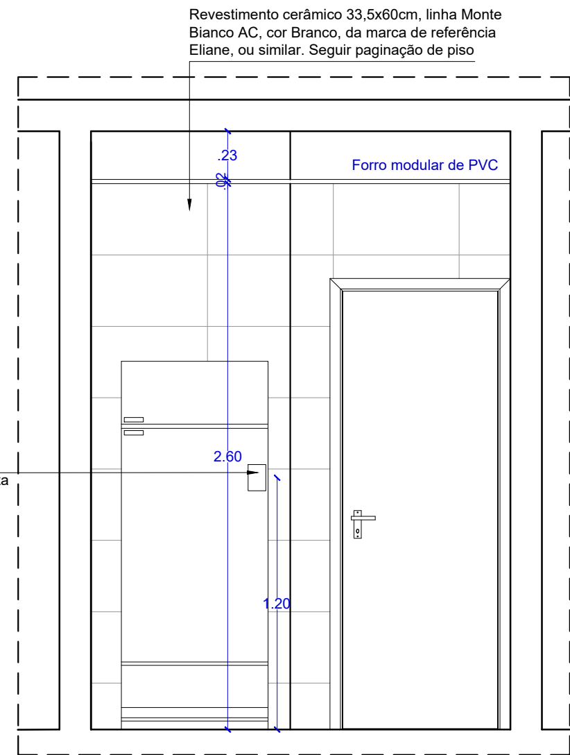
VISTA 02 COPA 1º PAV. ESCALA.....1/25
