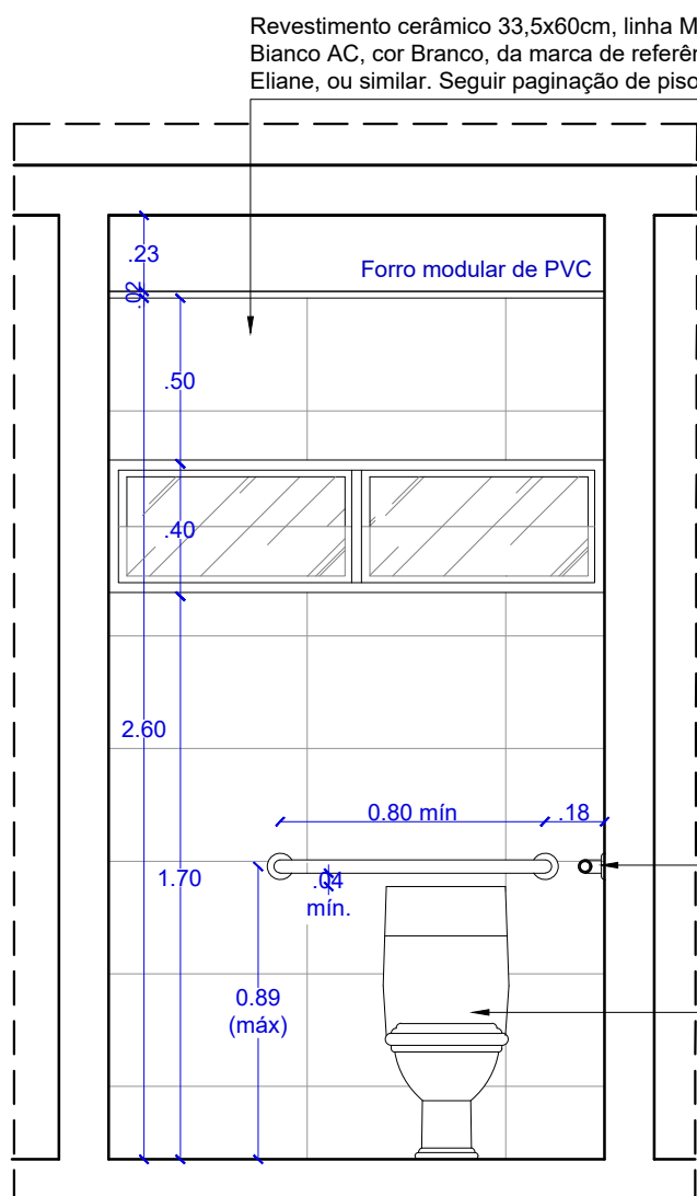
VISTA 03 WC PCD 1  PAV. ESCALA.....1/25
