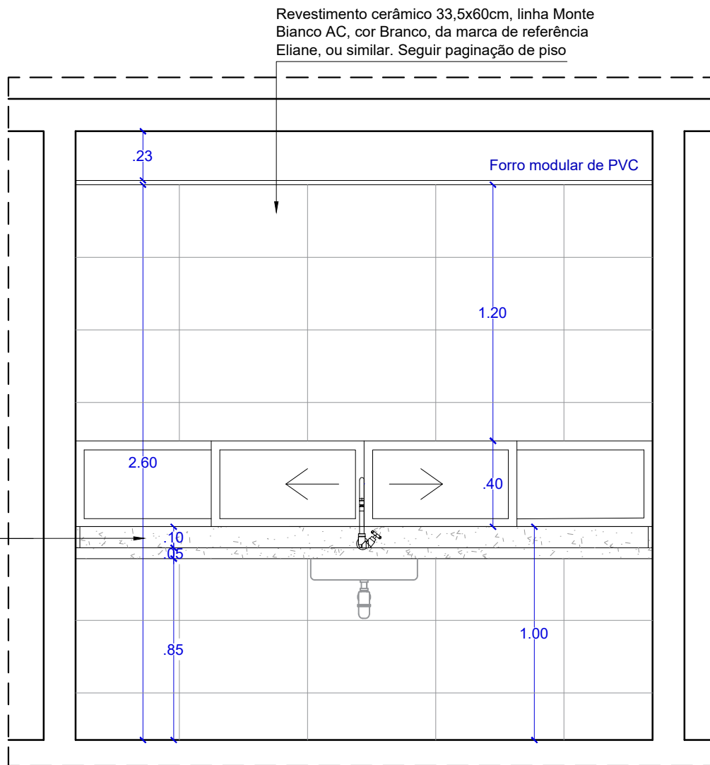
VISTA 02 COPA 1º PAV. ESCALA.....1/25
