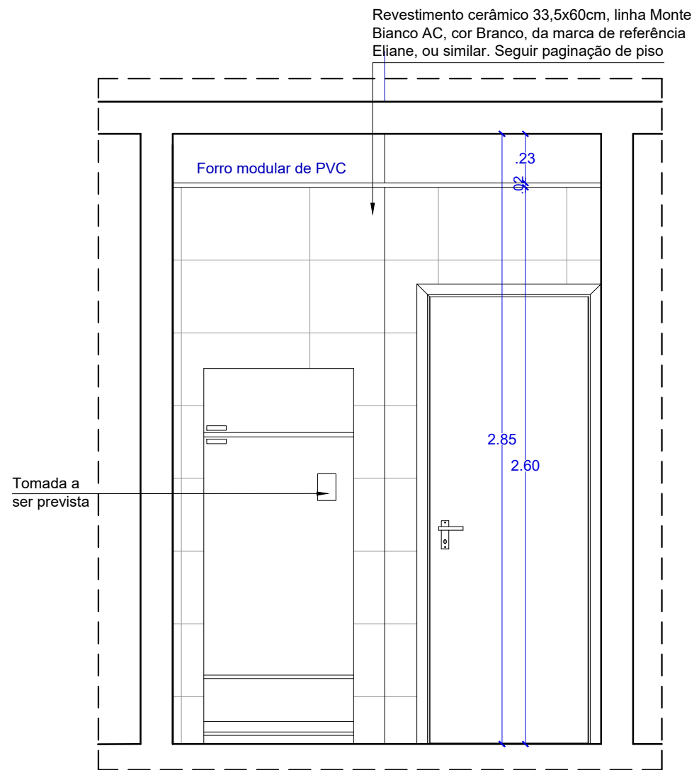
VISTA 02 COPA TÉRREO ESCALA.....1/25
