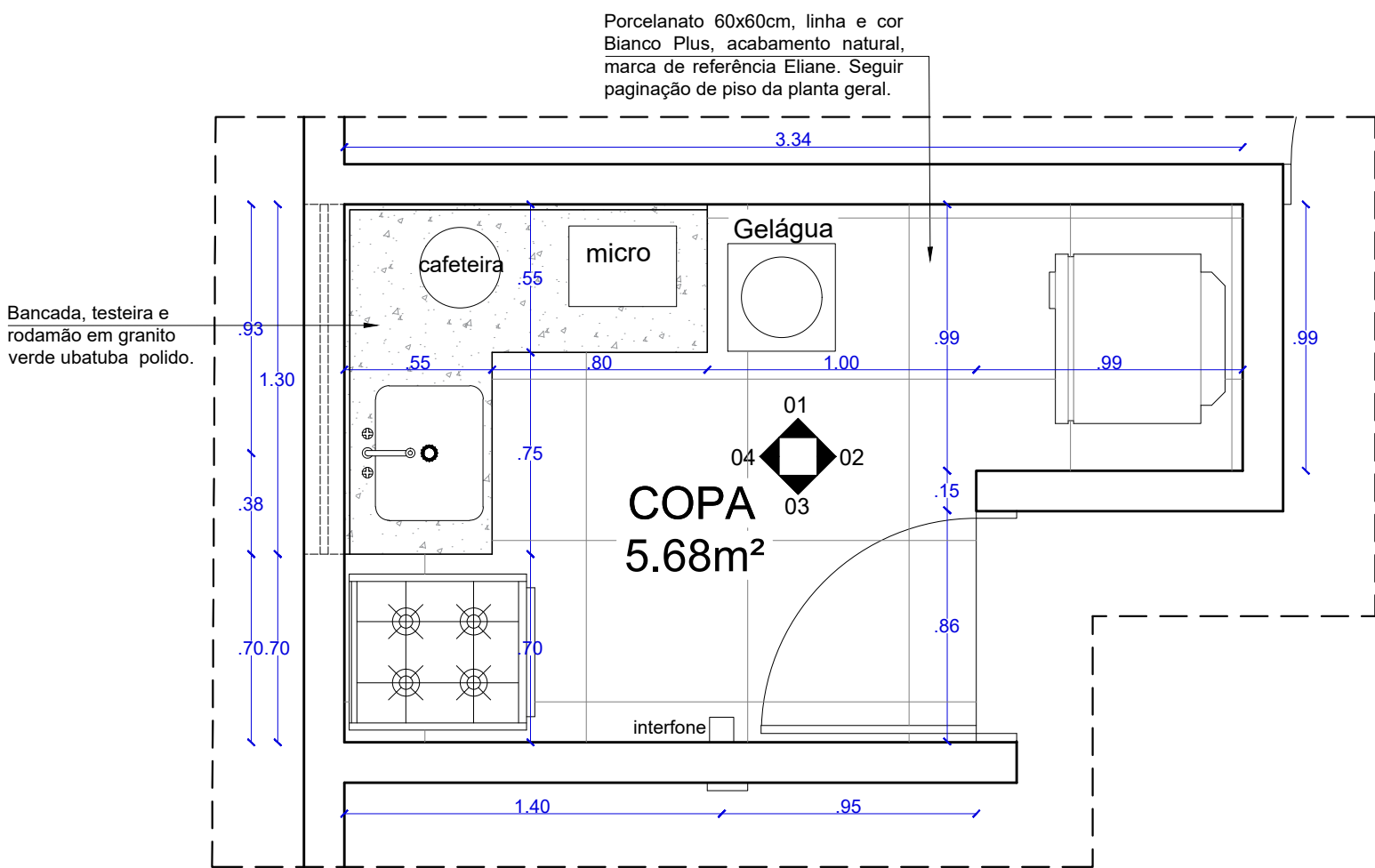
PLANTA BAIXA COPA TÉRREO ESCALA.....1/25
