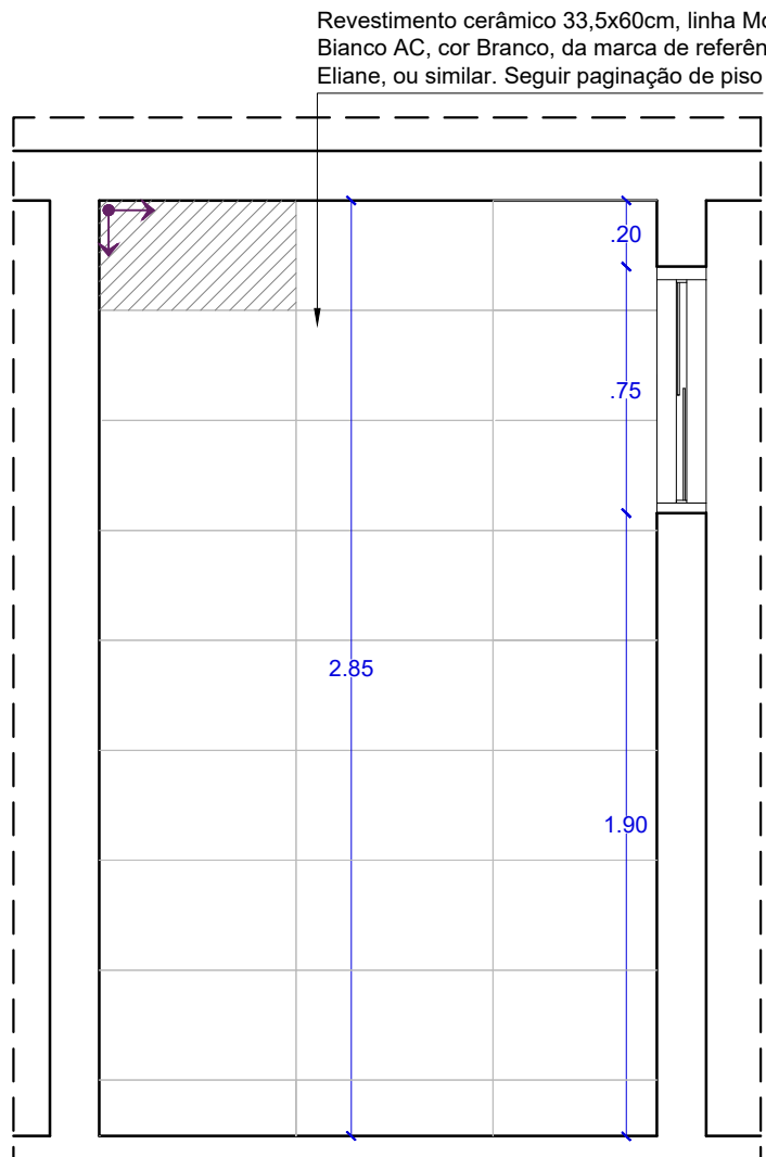
VISTA 01 WC DML ESCALA.....1/25
