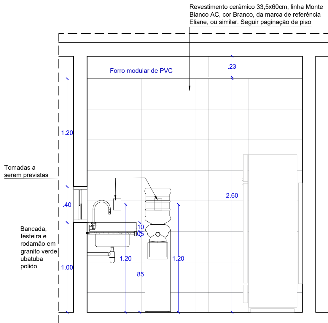
VISTA 03 COPA 1º PAV. ESCALA.....1/25
