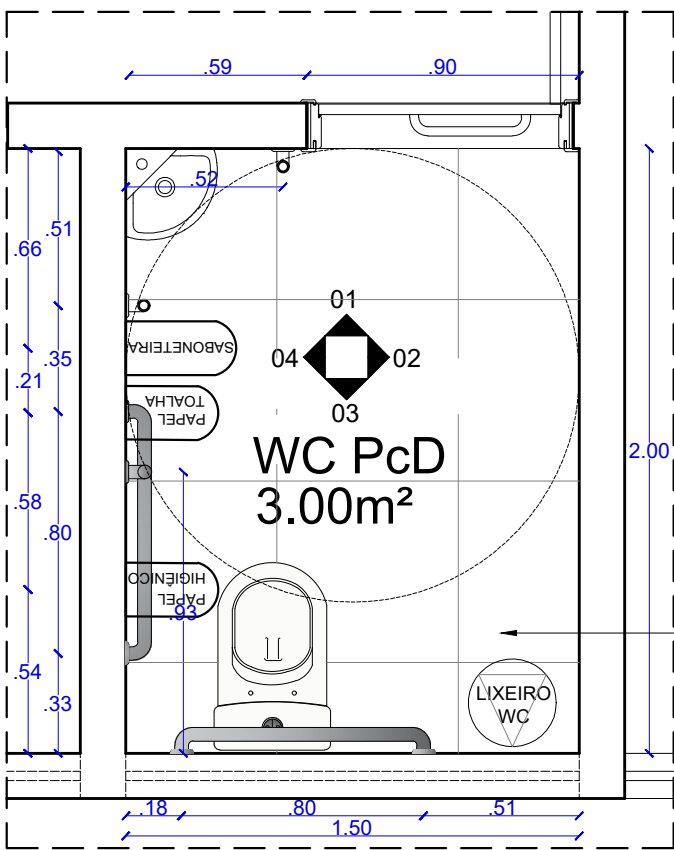
PLANTA BAIXA WC PCD 1  PAV. ESCALA.....1/25
