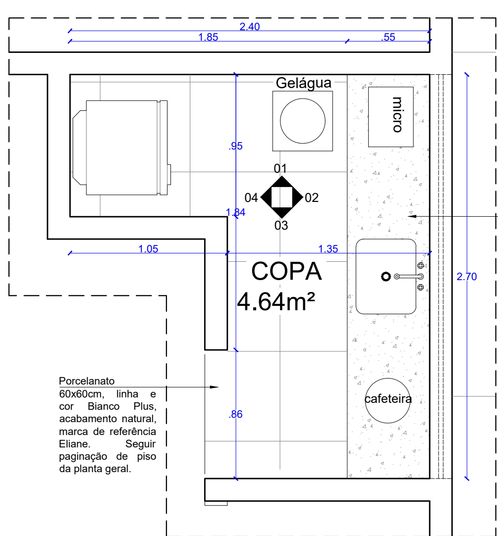
PLANTA BAIXA COPA DIREITA 1º PAV. ESCALA.....1/25
