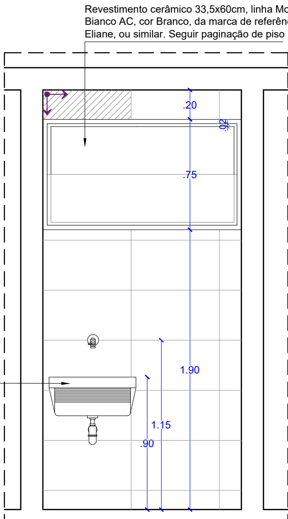
VISTA 02 WC DML ESCALA.....1/25
