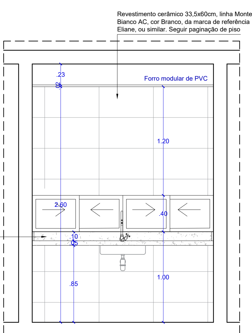
VISTA 04 COPA 1º PAV. ESCALA.....1/25
