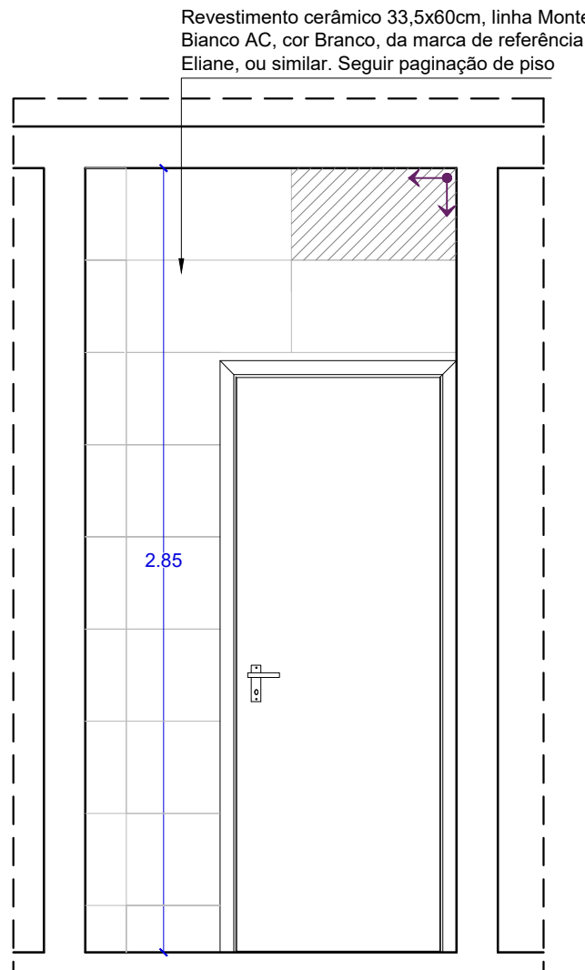
VISTA 04 WC DML ESCALA.....1/25
