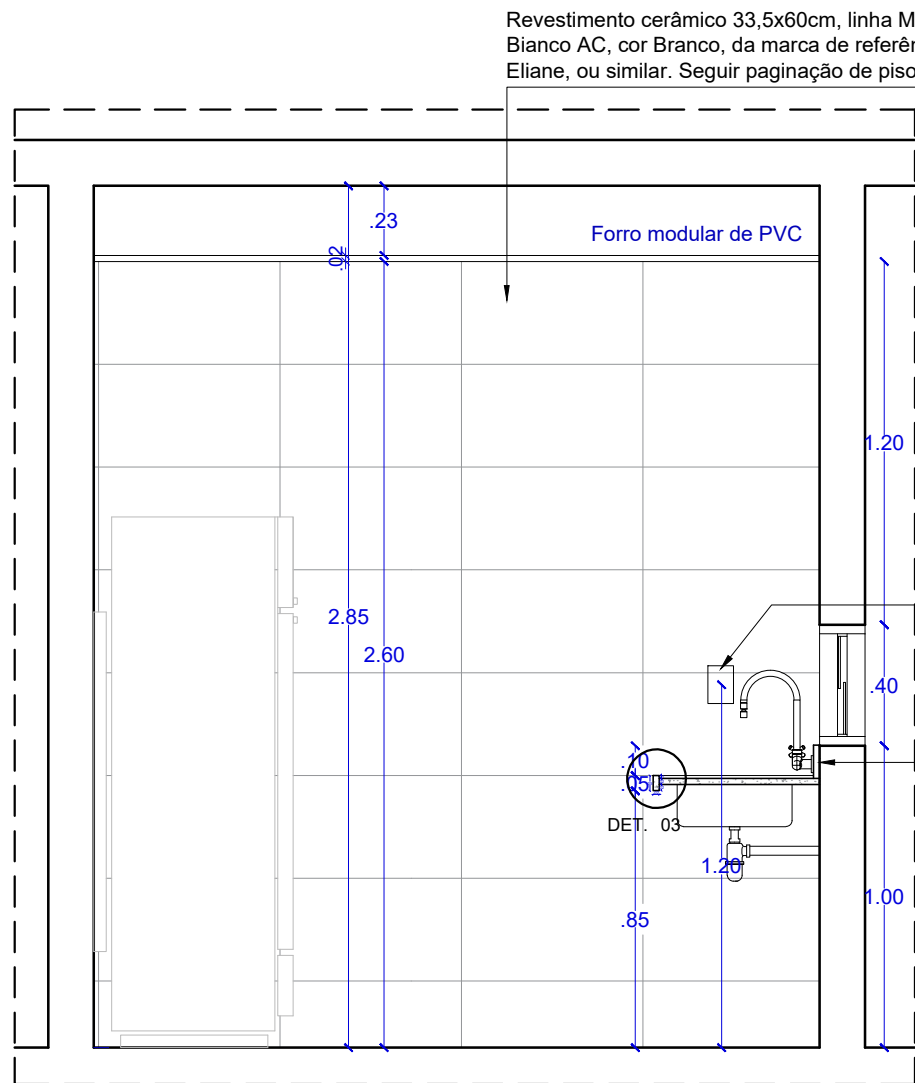
VISTA 01 COPA 1º PAV. ESCALA.....1/25
