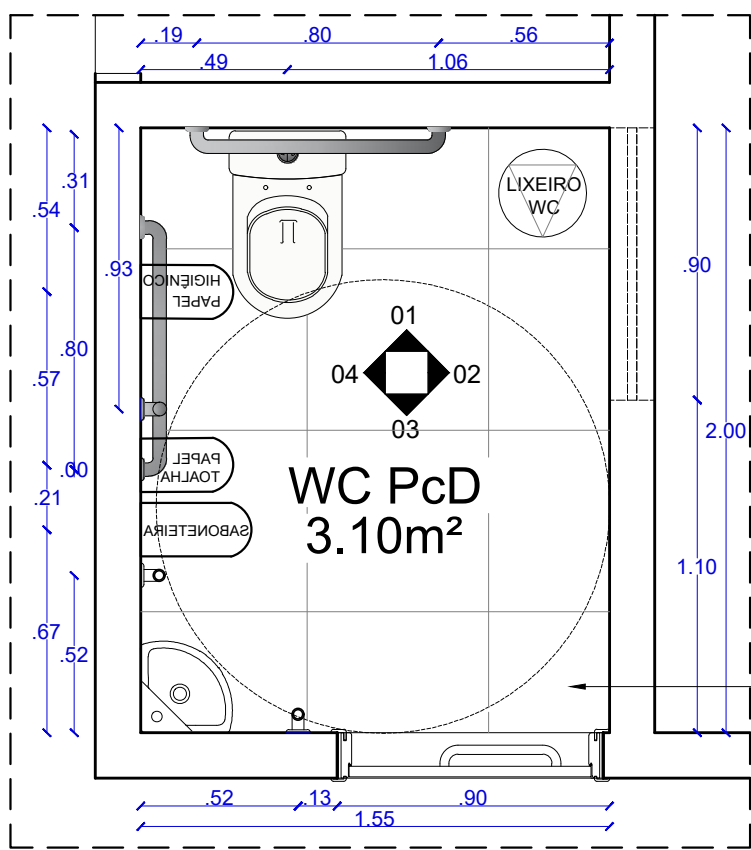
PLANTA BAIXA WC PCD T RREO ESCALA.....1/25
