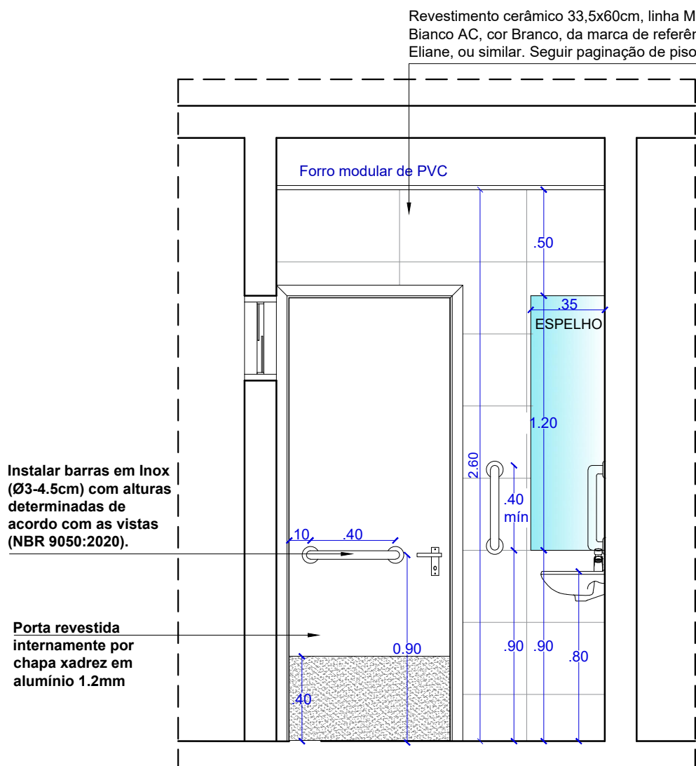
VISTA 03 WC PCD T RREO ESCALA.....1/25
