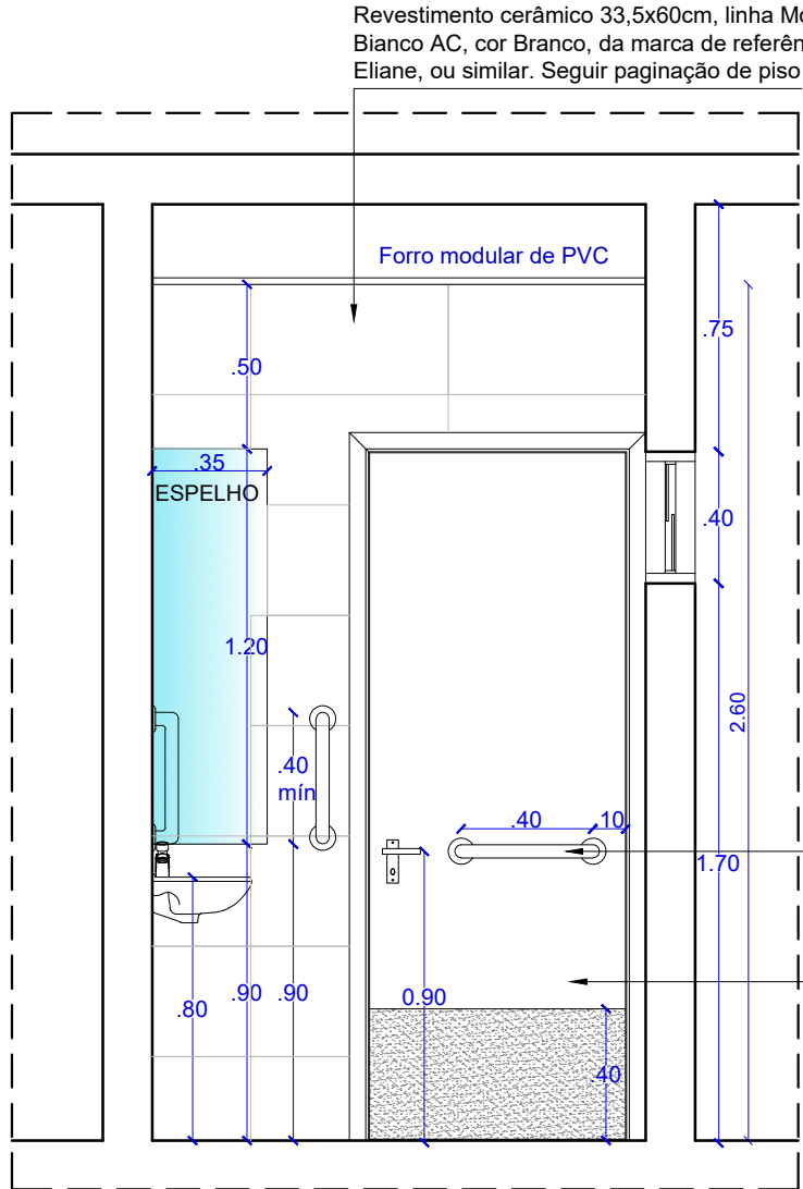
VISTA 01 WC PCD 1  PAV. ESCALA.....1/25
