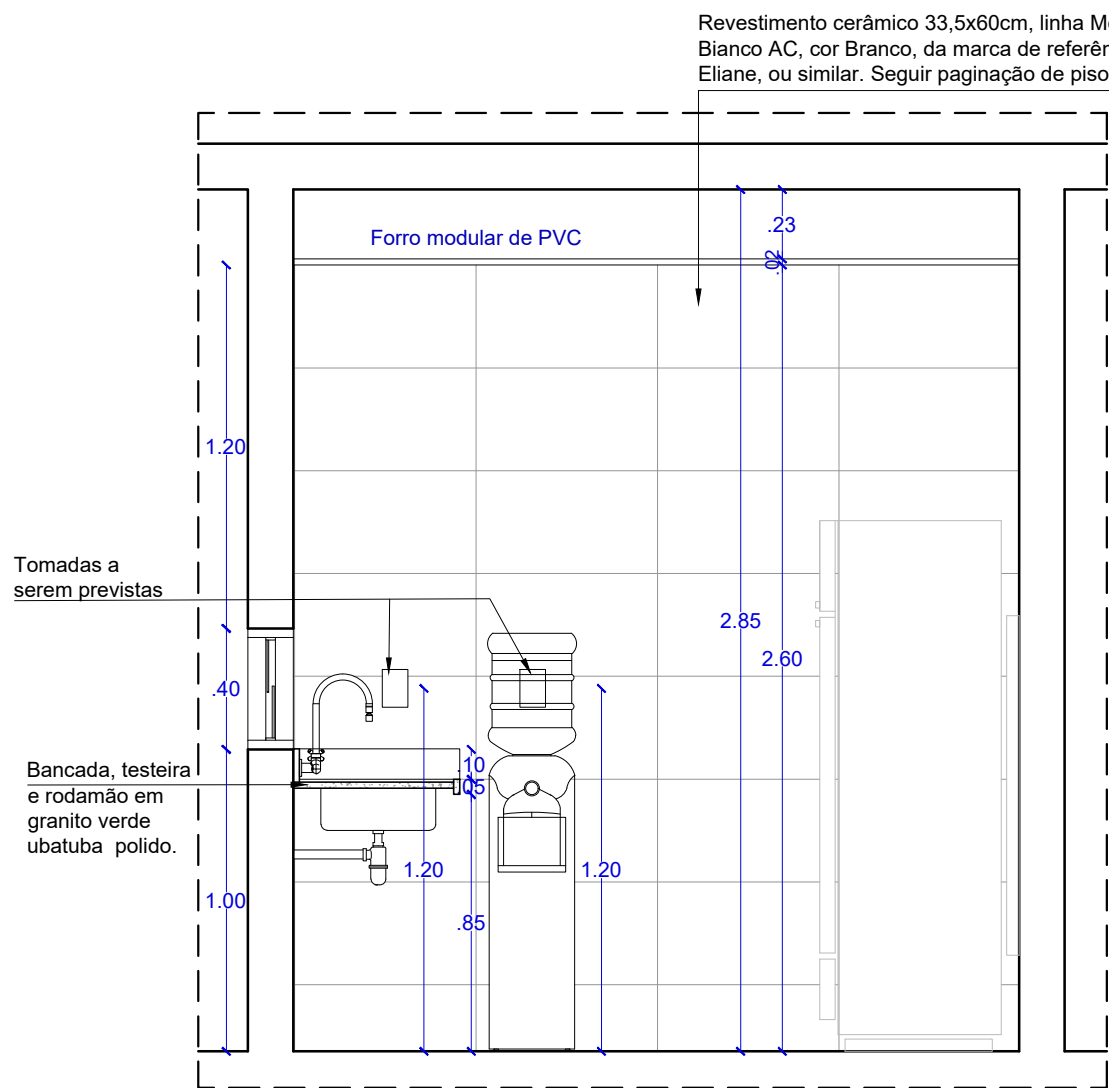
VISTA 01 COPA 1º PAV. ESCALA.....1/25
