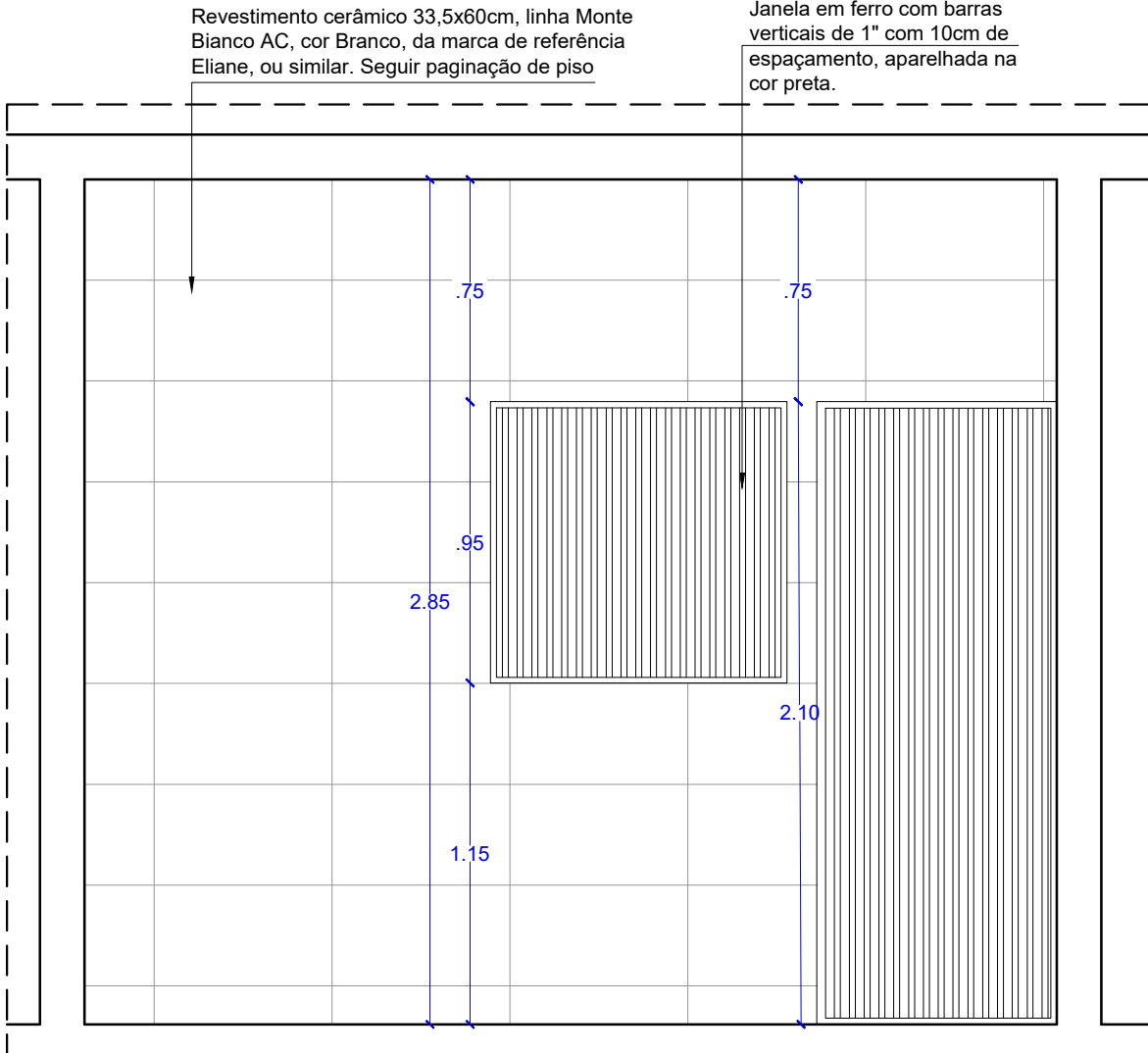
VISTA 02 CELTA ESCALA.....1/25
