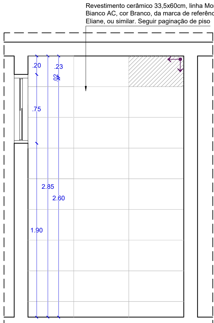
VISTA 03 WC DML ESCALA.....1/25
