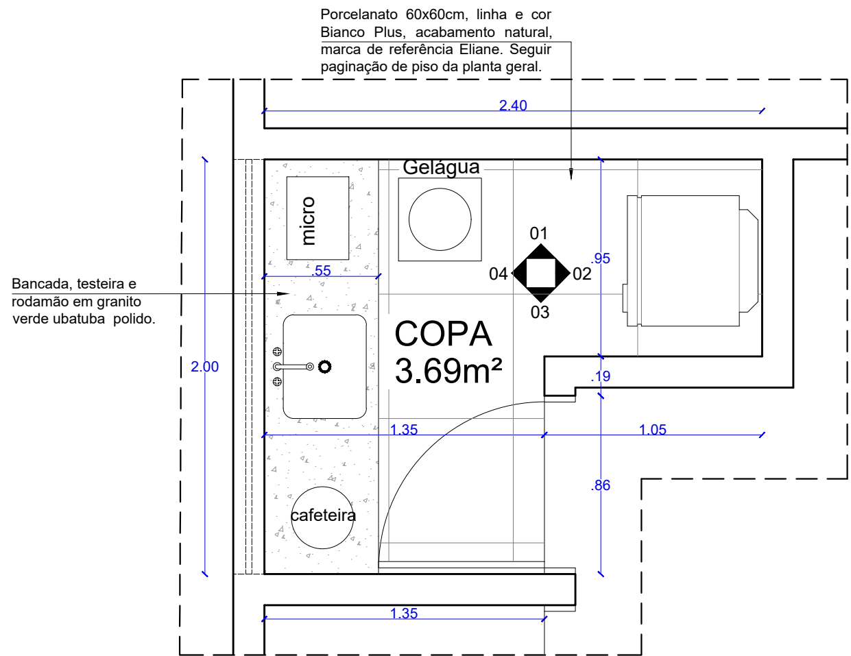
PLANTA BAIXA COPA ESQUERDA 1º PAV. ESCALA.....1/25
