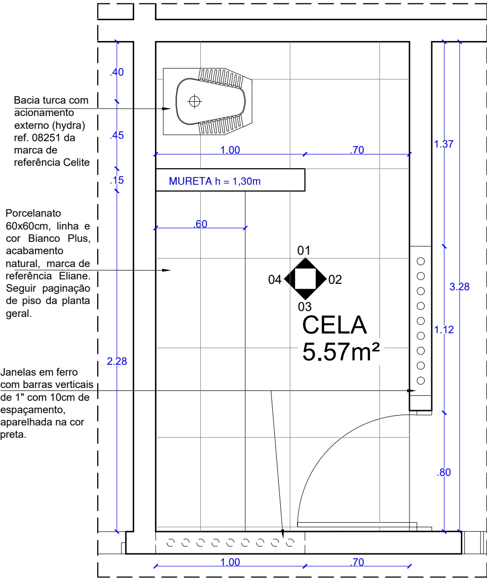
PLANTA BAIXA CELTA ESCALA.....1/25
