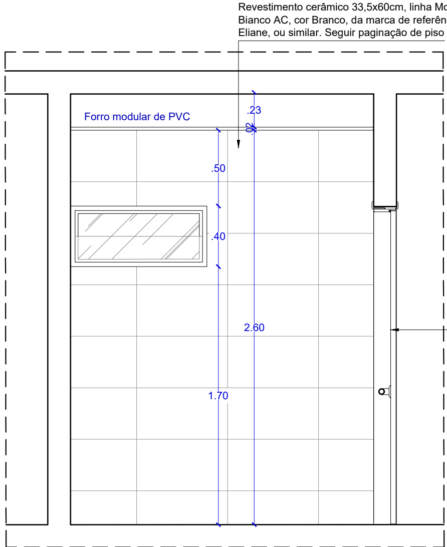
VISTA 02 WC PCD T RREO ESCALA.....1/25
