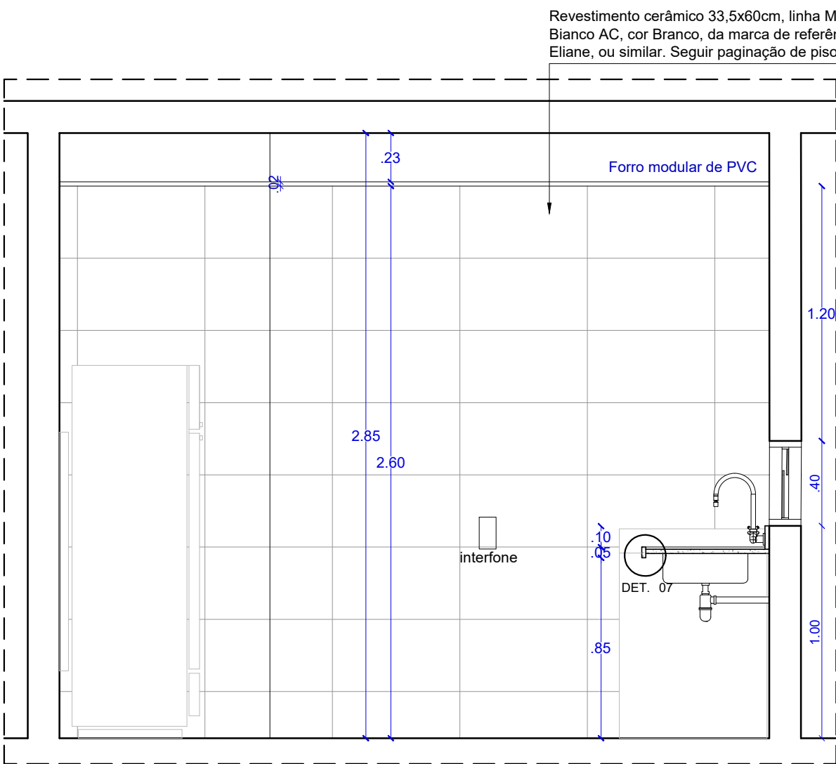
VISTA 03 COPA TÉRREO ESCALA.....1/25
