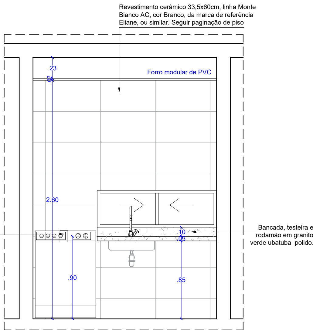
VISTA 04 COPA TÉRREO ESCALA.....1/25
