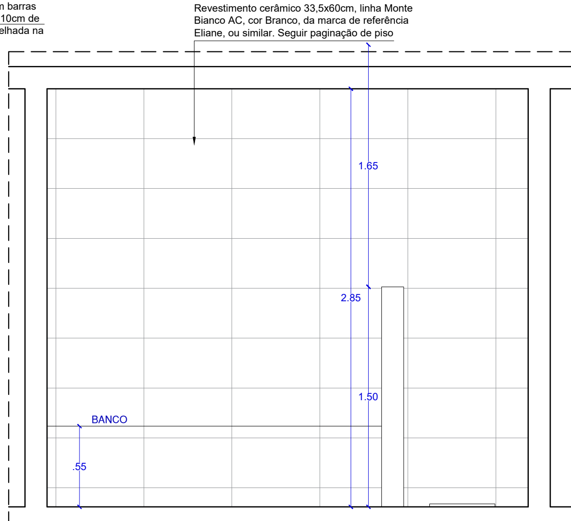
VISTA 04 CELTA ESCALA.....1/25
