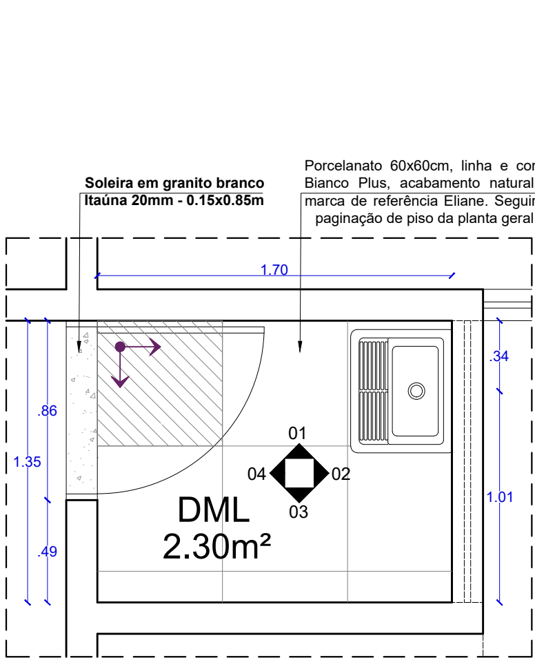
PLANTA BAIXA DML ESCALA.....1/25
