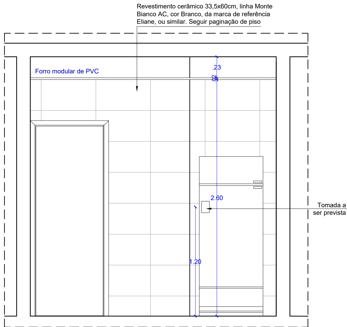
VISTA 04 COPA 1º PAV. ESCALA.....1/25
