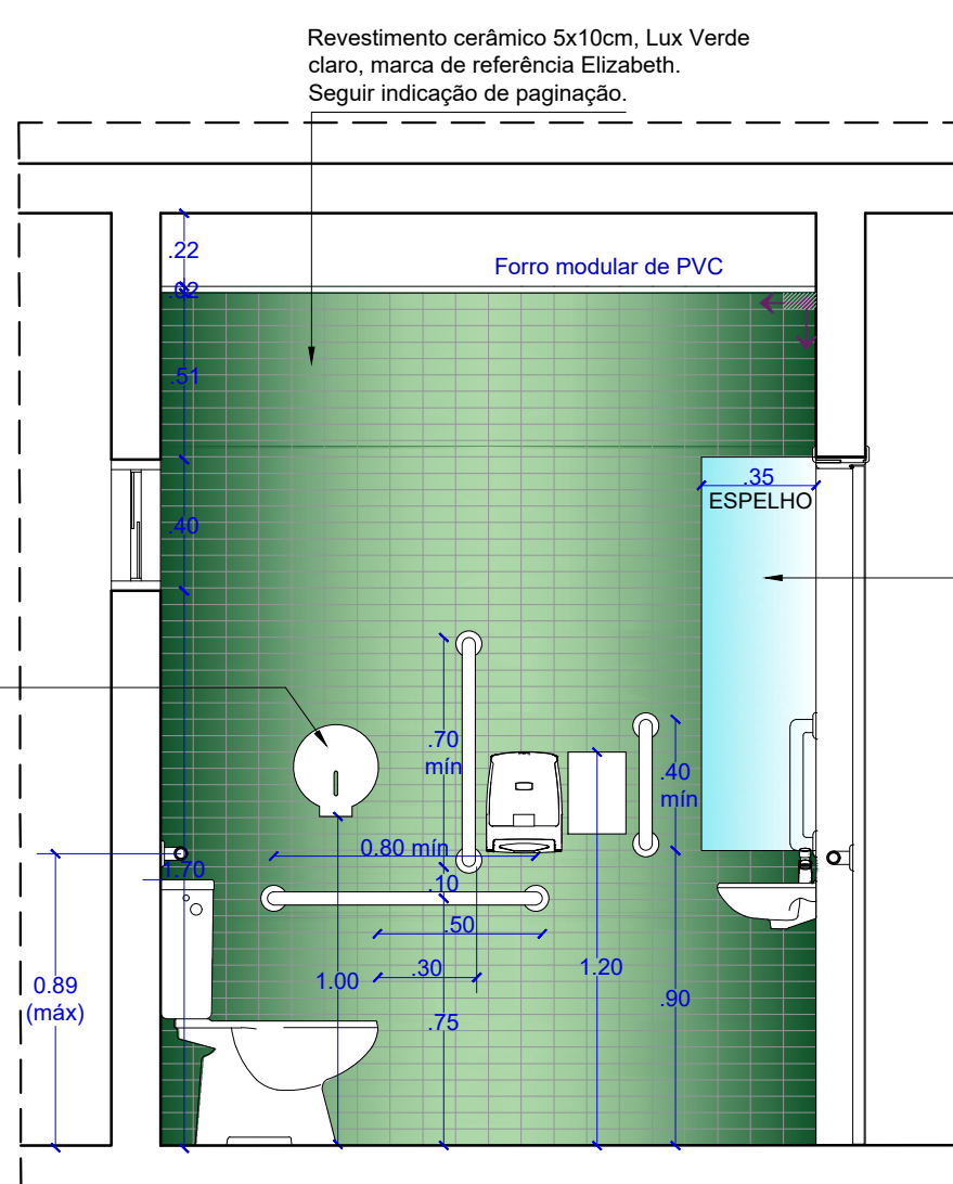
VISTA 04 WC PCD 1  PAV. ESCALA.....1/25
