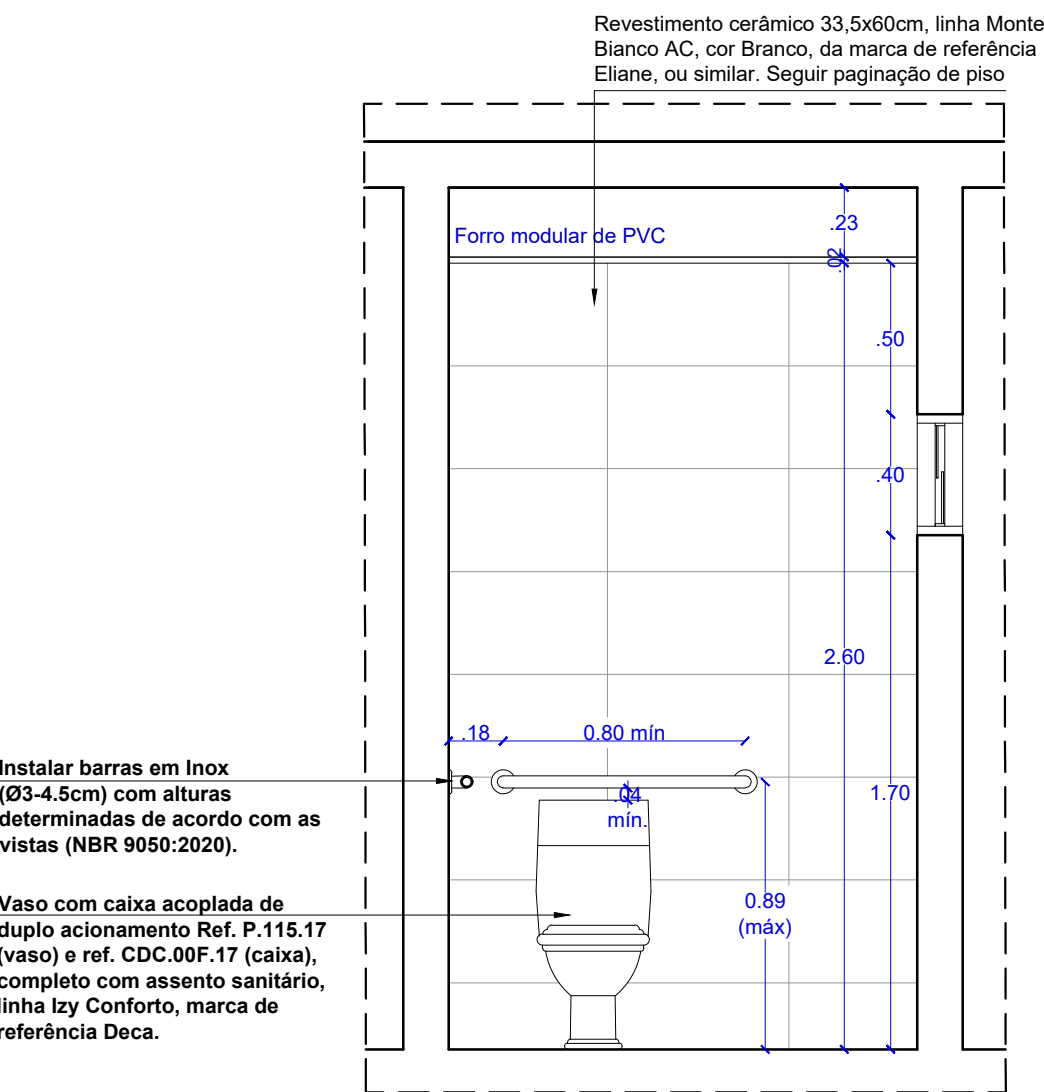
VISTA 01 WC PCD T RREO ESCALA.....1/25
