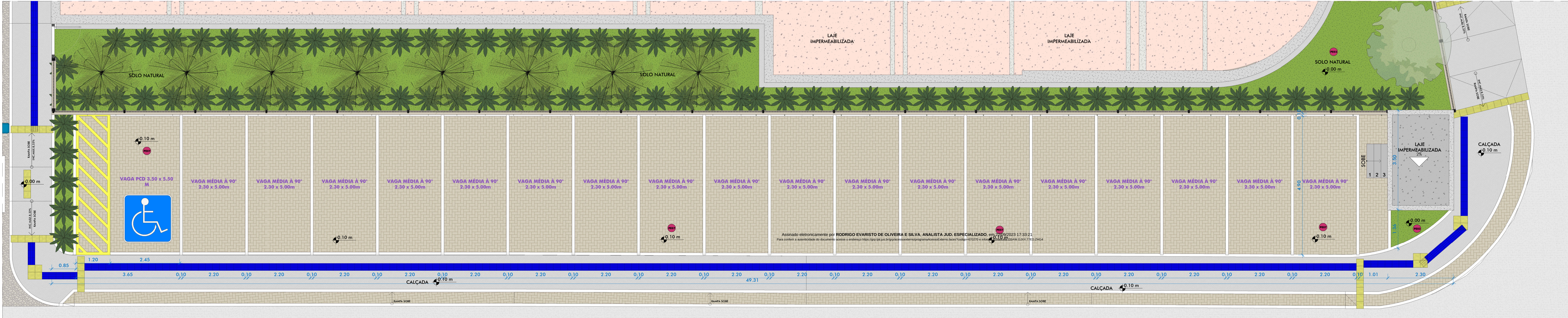
DETALHE 02 - PB AGENCIAMENTO 06 ESC: 1:50
