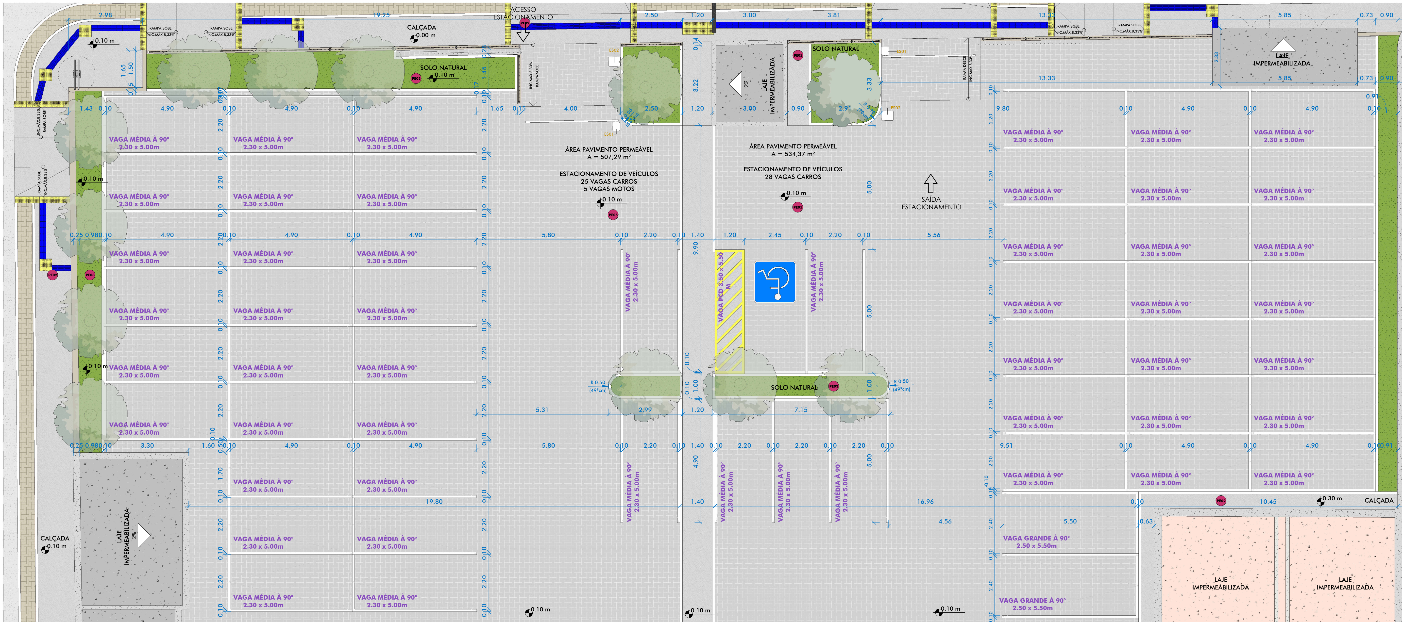
DETALHE 03 - PB AGENCIAMENTO 07 ESC: 1:75
