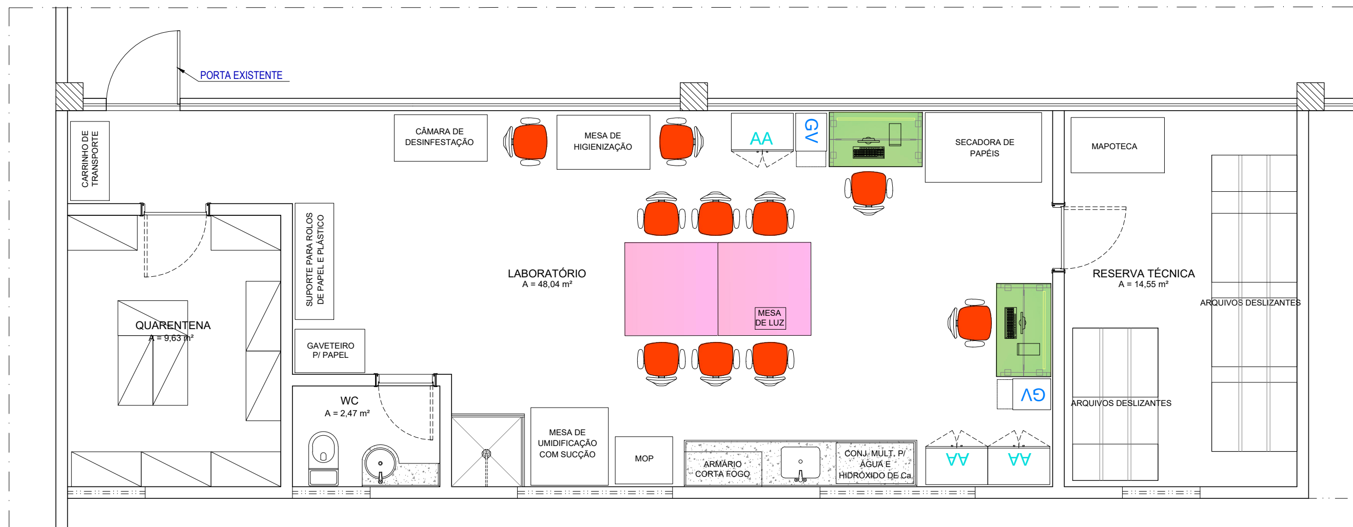
PLANTA BAIXA ESCALA.....1/50
