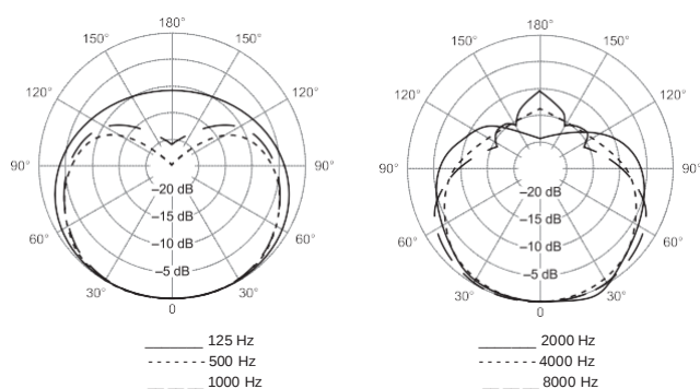
Padrão Polar Medido em 1000 Hz
