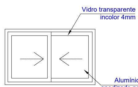
ELEVÇÃO JANELA ALTA ESCALA.....1/25
