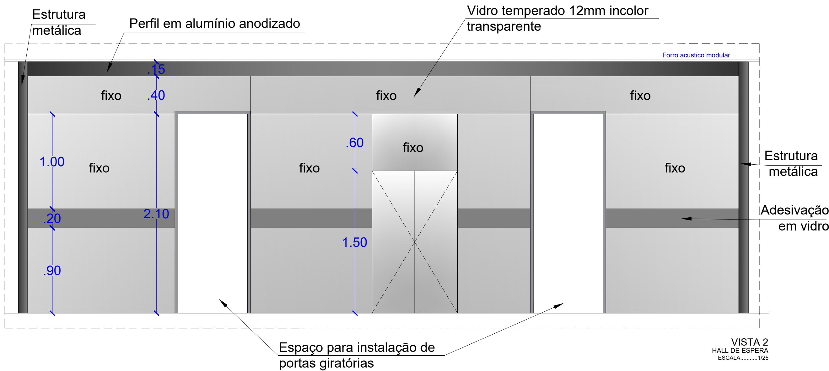
VISTA 1 HALL DE ESPERA ESCALA.....1/25
