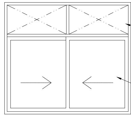
ELEVÇÃO ESQUADRIA ALUM. E VIDRO ESCALA.....1/25
