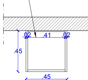
PLANTA BAIXA ESCALA.....1/25
