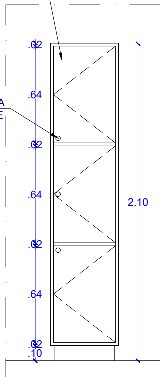
ELEV. 01 - COM PORTAS ESCALA.....1/25
