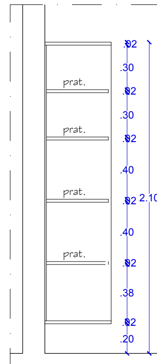
CORTE TRANSVERSAL ESCALA.....1/25
