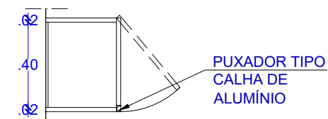
CORTE TRANSVERSAL ESCALA.....1/25
