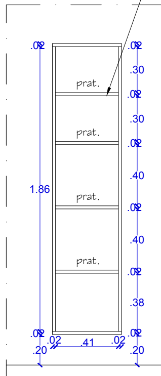
ELEVação FRONTAL ESCALA.....1/25
