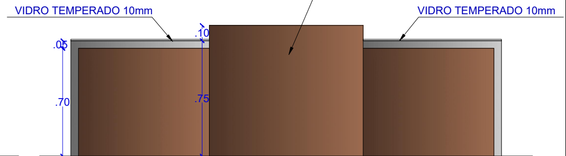
VISTA 02 - BANCADA PRINCIPAL ESCALA.....1/25
