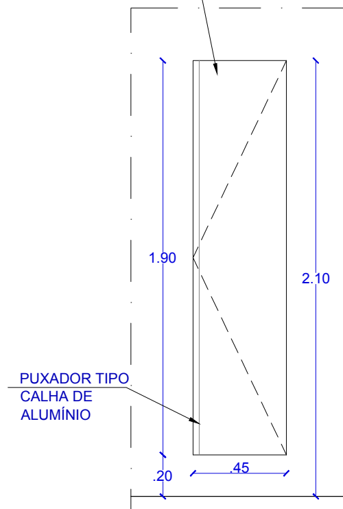
ELEV. 01 - COM PORTAS ESCALA.....1/25
