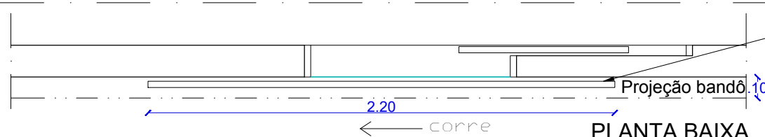
PLANTA BAIXA ESCALA.....1/25
