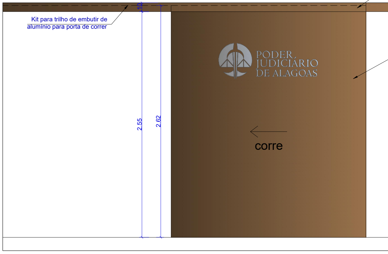
ELEVAÇÃO FRONTAL ESCALA.....1/25
