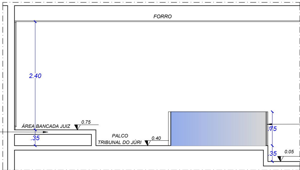
CORTE BB' DETALHE - GUARDA CORPO TRIBUNAL DO JÚRI ESCALA.....1/25
