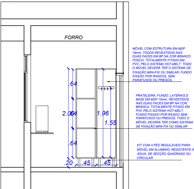
VISTA 02 - ÁREA DE SERVIÇO PORTAS ABERTAS ESCALA ..... 1/50
