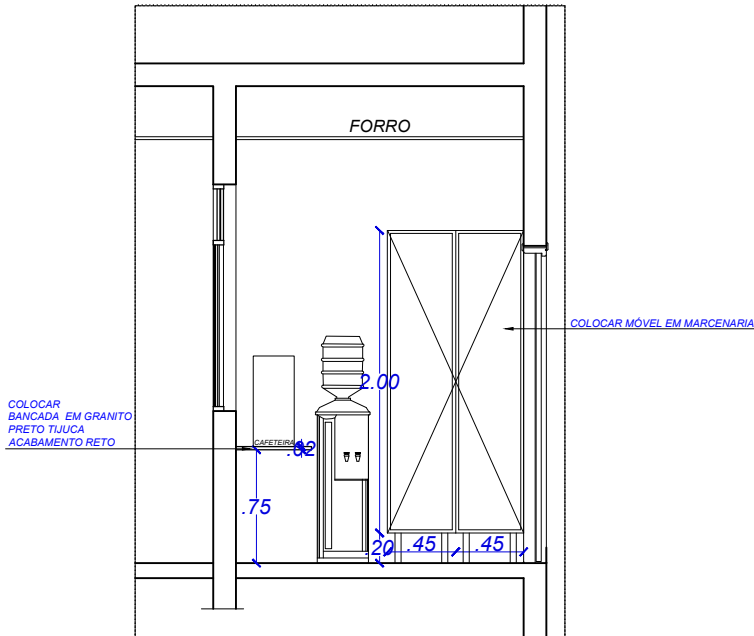
VISTA 02 - ÁREA DE SERVIÇO PORTAS FECHADAS ESCALA ..... 1/50
