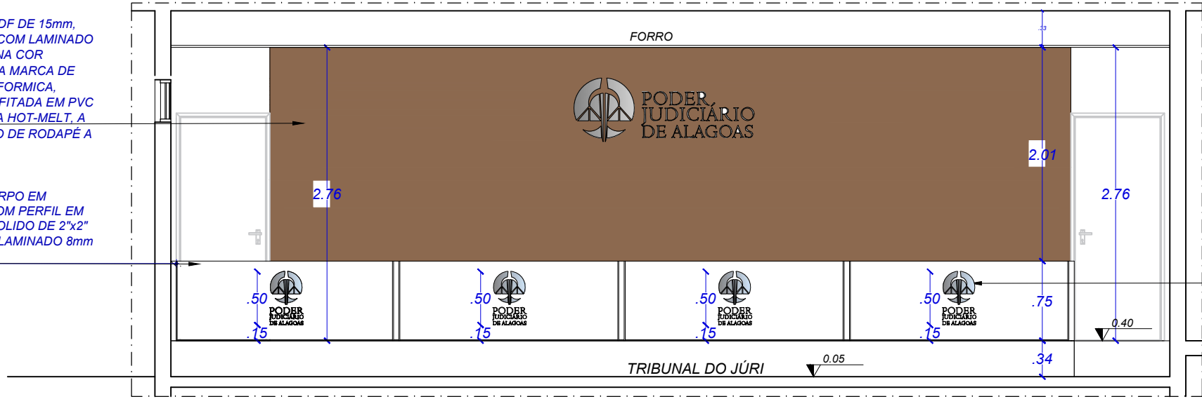
CORTE AA' DETALHE - GUARDA CORPO TRIBUNAL DO JÚRI ESCALA.....1/25
