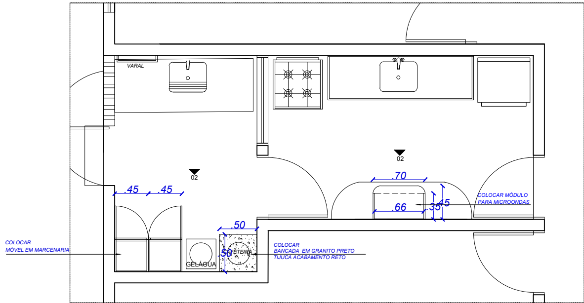
PLANTA BAIXA -COZINHA E ÁREA DE SERVIÇO ESCALA ..... 1/50
