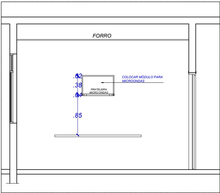
VISTA 01 - COZINHA ESCALA ..... 1/50
