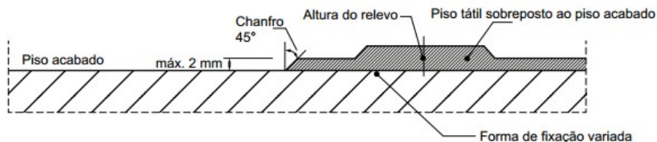
DETALHE DE APLICAÇÃO DO PISO TÁTIL
