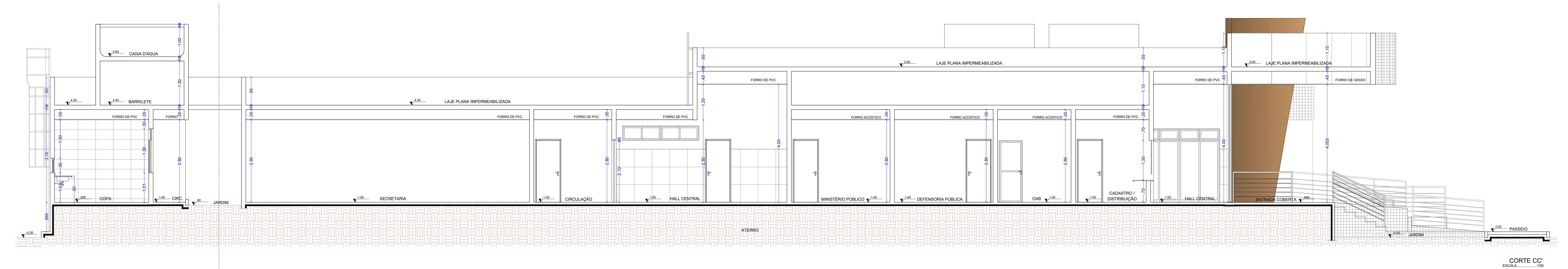
CORTE CC' ESCALA 1:100
