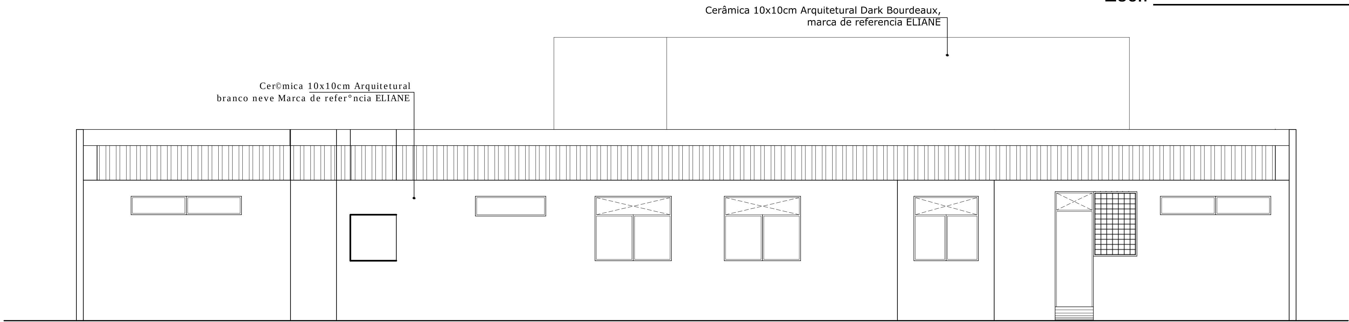
FACHADA POSTERIOR Esc.: 1/50
