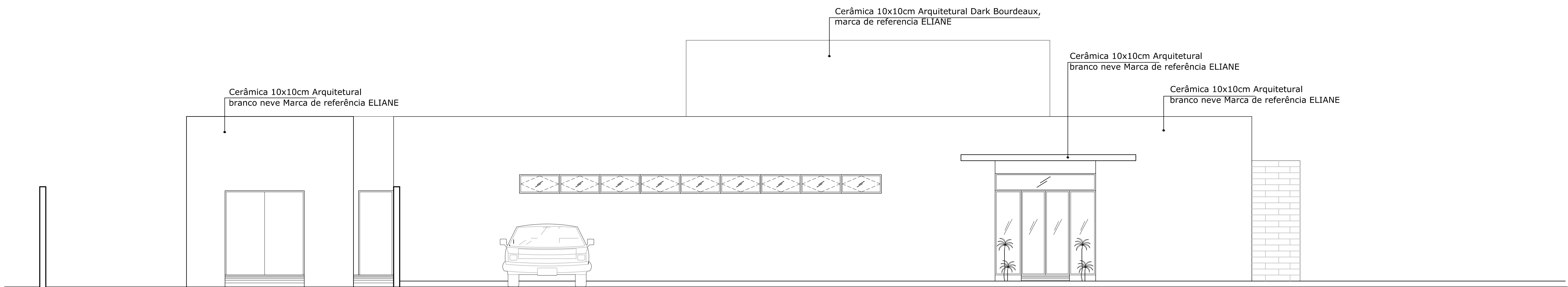
FACHADA LATERAL ESQUERDA Esc____1/50
