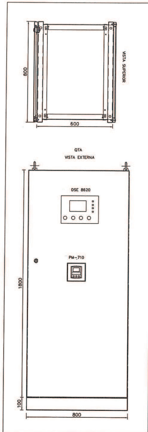
DETALHE DO QTA (QUADRO DE TRANSFERÊNCIA AUTOMÁTICA) SEM ESCALA MEDIDAS EM MM
