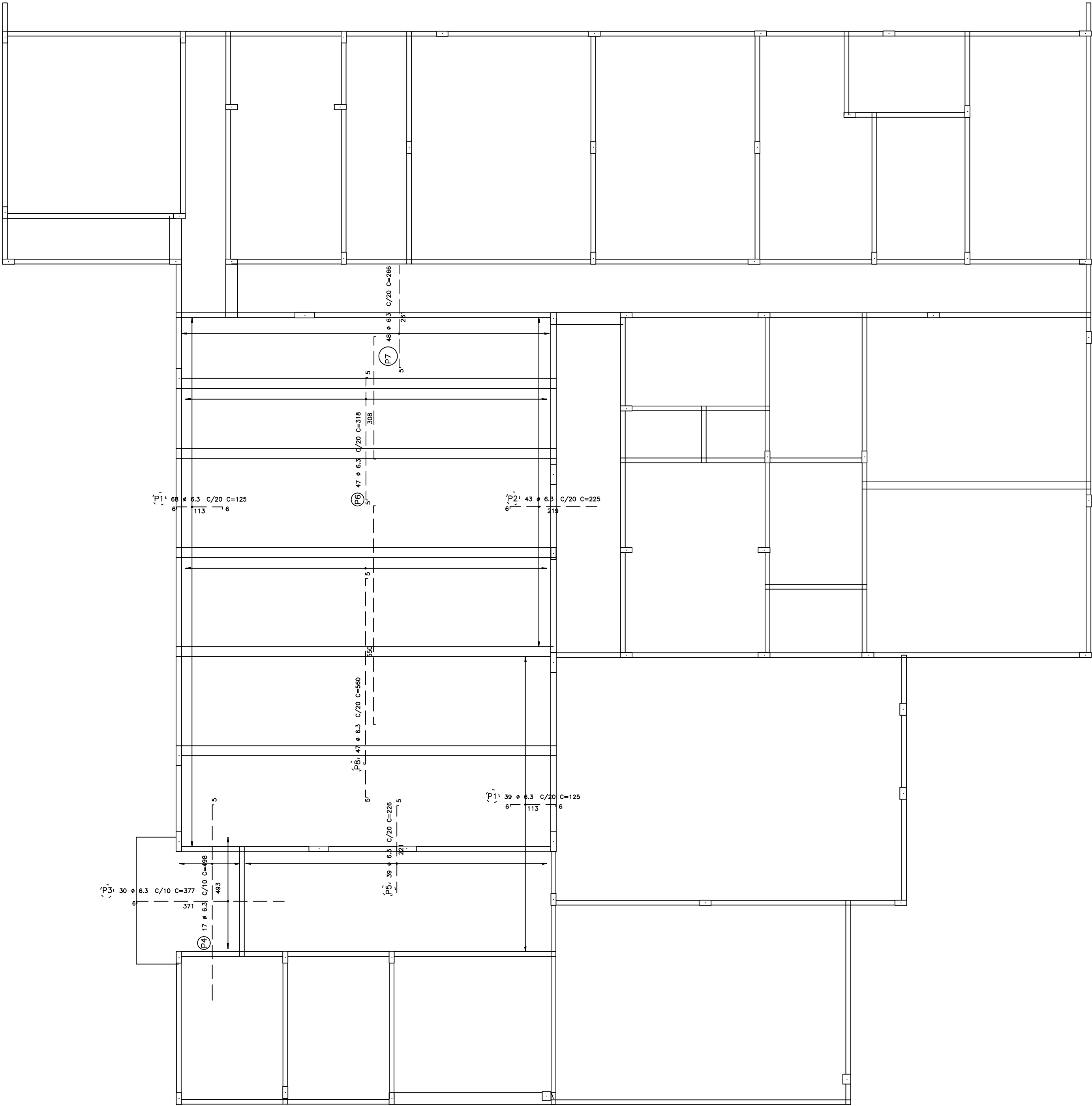
Coberta – Armadura negativa 1X
