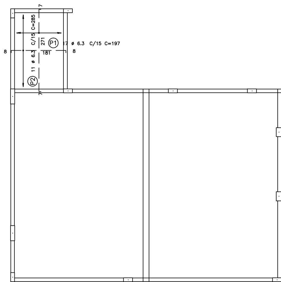
Laje caixa água – Armadura negativa
