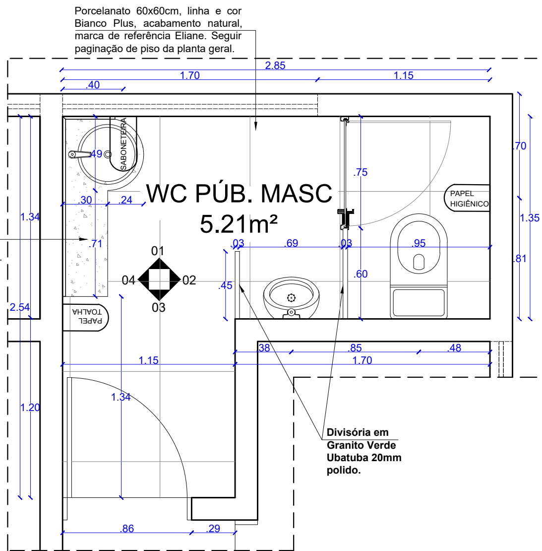
PLANTA BAIXA WC PUB. MASCULINO TÉRREO ESCALA.....1/25
