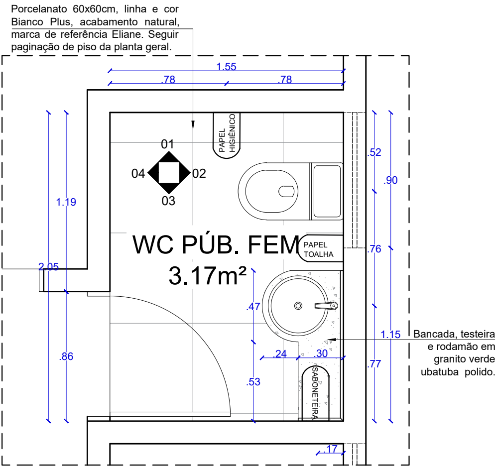
PLANTA BAIXA WC PUB. FEMININO TÉRREO ESCALA.....1/25
