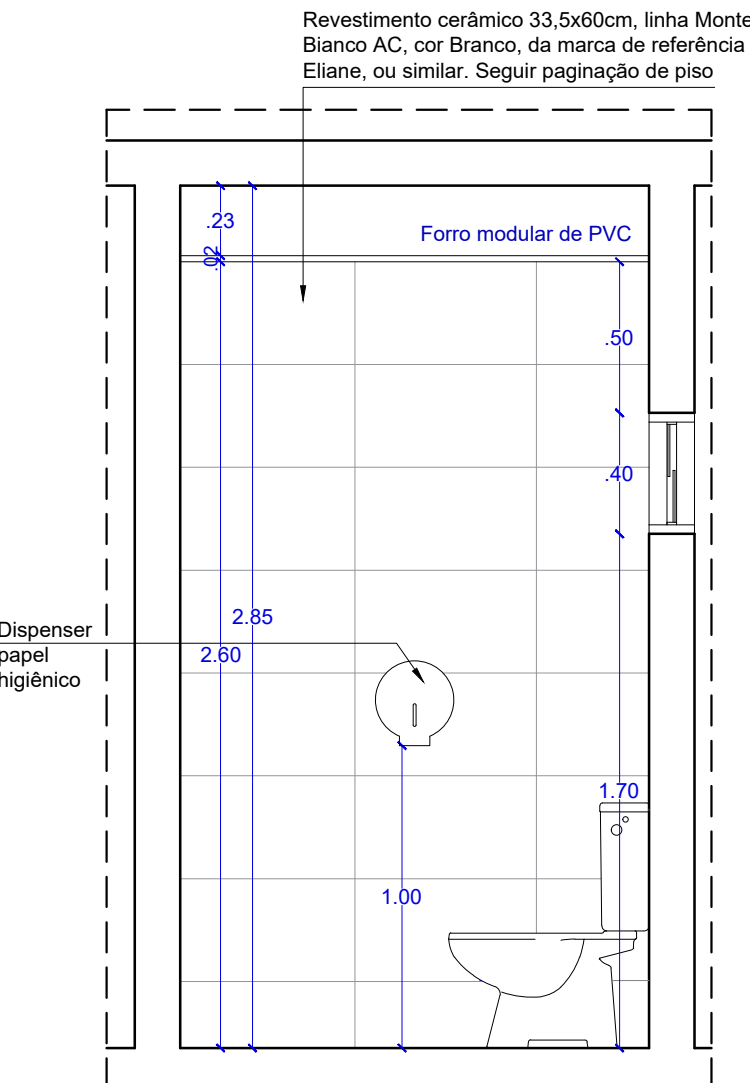
VISTA 01 WC PUB. FEMININO TÉRREO ESCALA.....1/25
