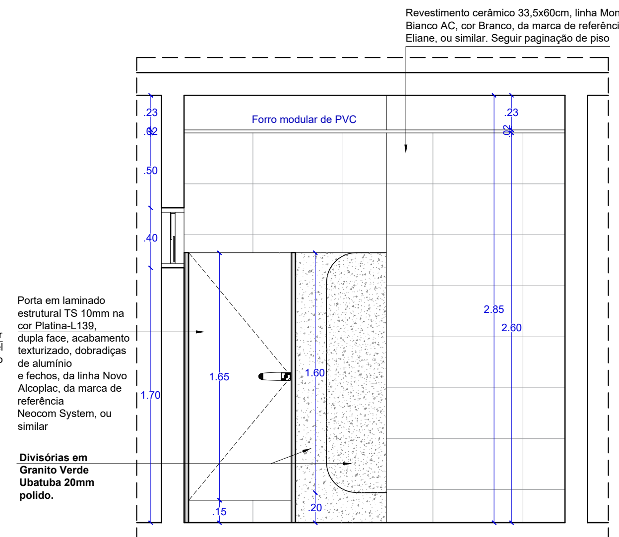
VISTA 02 WC PUB. MASCULINO TÉRREO ESCALA.....1/25
