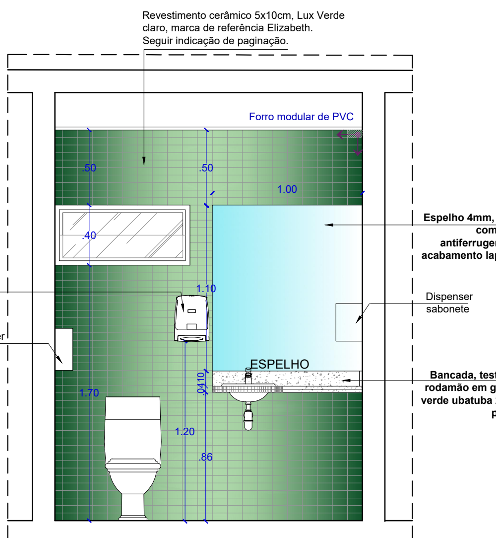
VISTA 02 WC PUB. FEMININO TÉRREO ESCALA.....1/25
