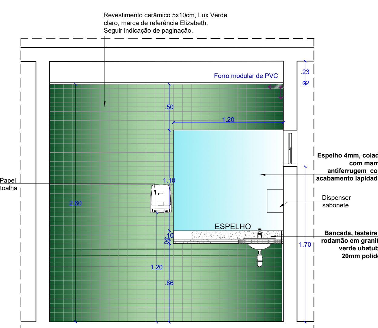
VISTA 04 WC PUB. MASCULINO TÉRREO ESCALA.....1/25
