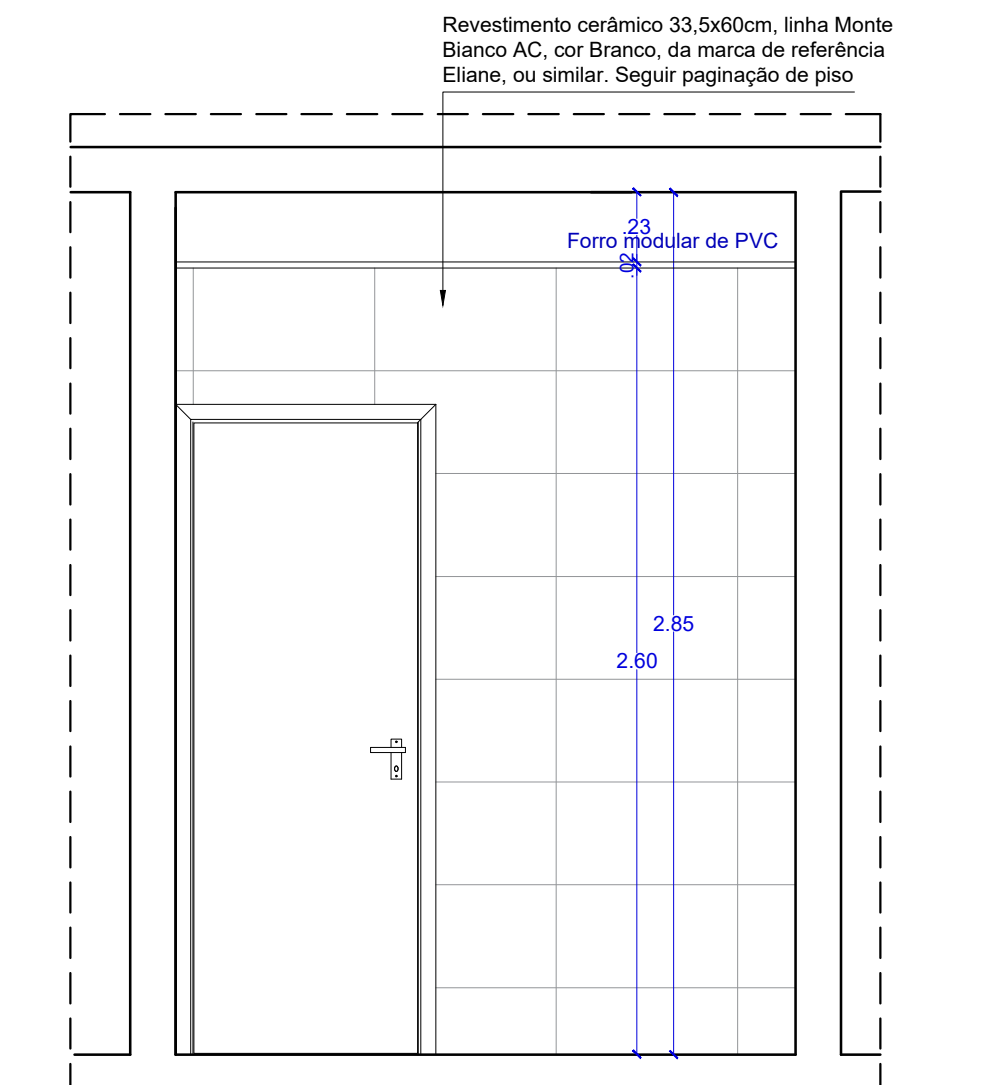
VISTA 04 WC PUB. FEMININO TÉRREO ESCALA.....1/25
