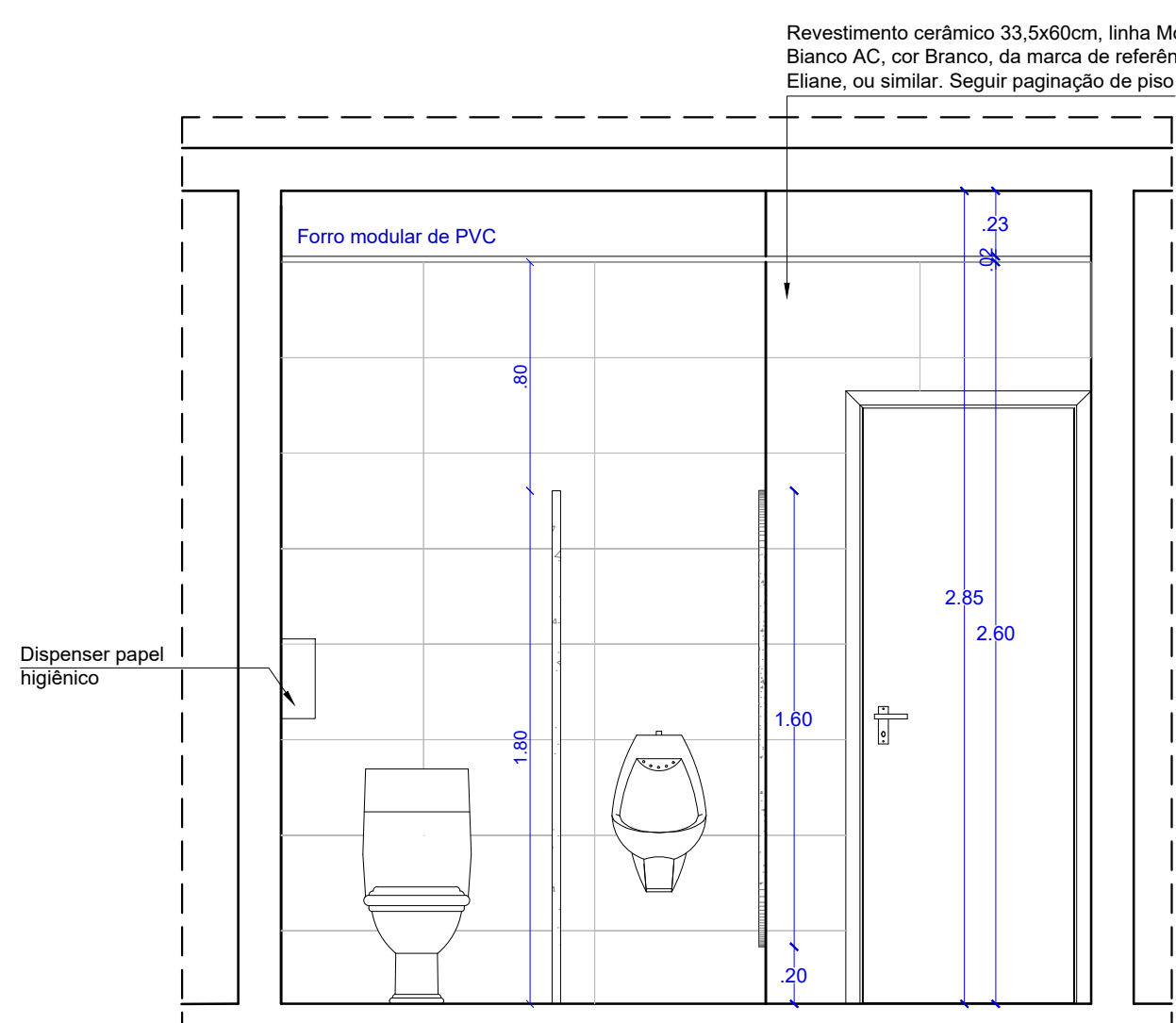
VISTA 03 WC PUB. MASCULINO TÉRREO ESCALA.....1/25
