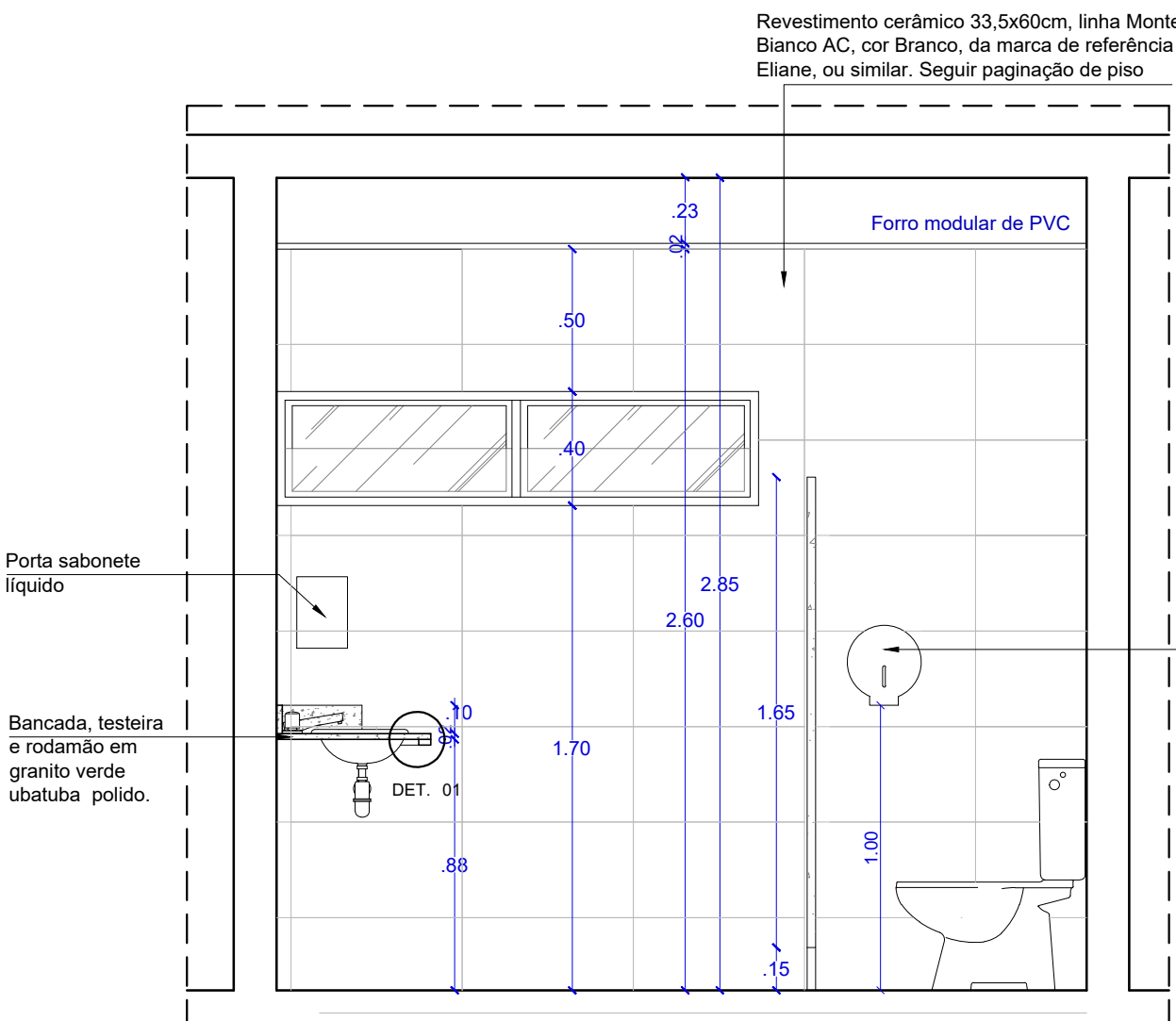
VISTA 01 WC PUB. MASCULINO TÉRREO ESCALA.....1/25
