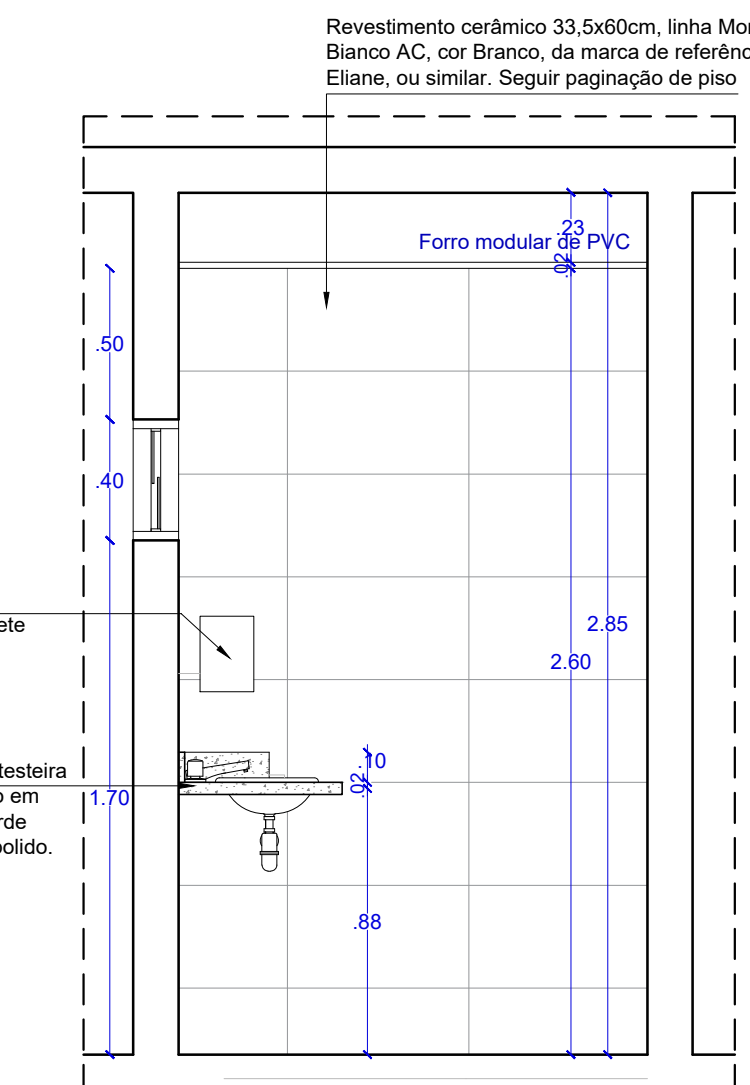
VISTA 03 WC PUB. FEMININO TÉRREO ESCALA.....1/25
