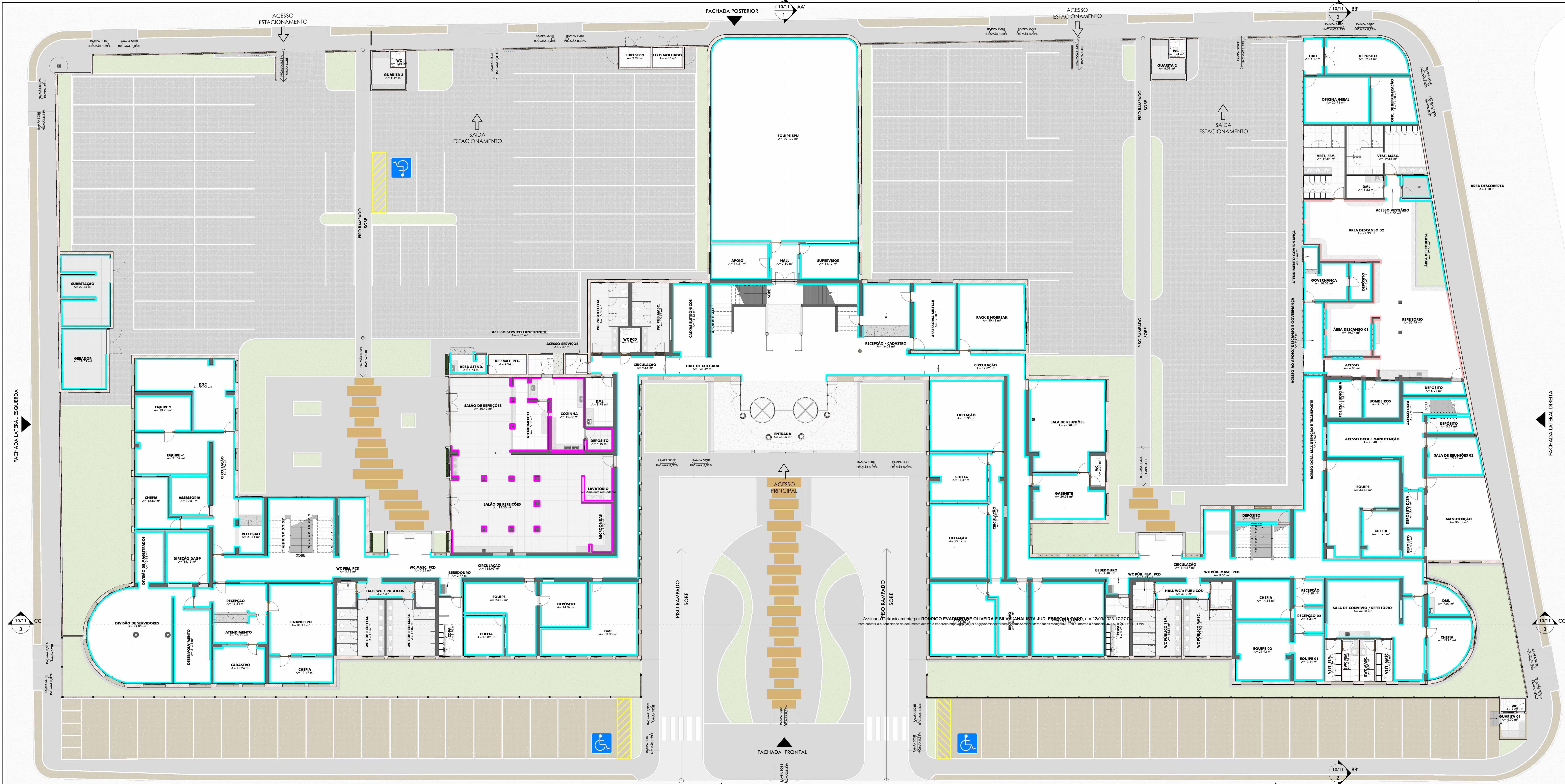
PB DE ESPECIFICAÇÃO DE RODAPÉS - TÉRREO ESC: 1 : 125
