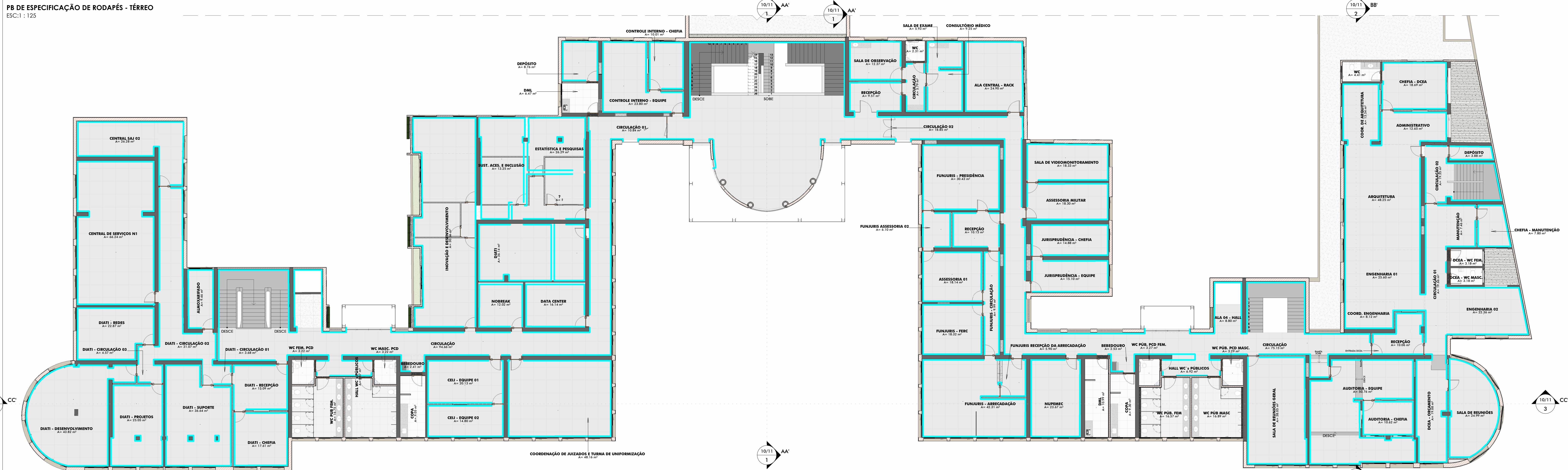
PB DE ESPECIFICAÇÃO DE RODAPÉS - 1º PAV. ESC: 1 : 125
