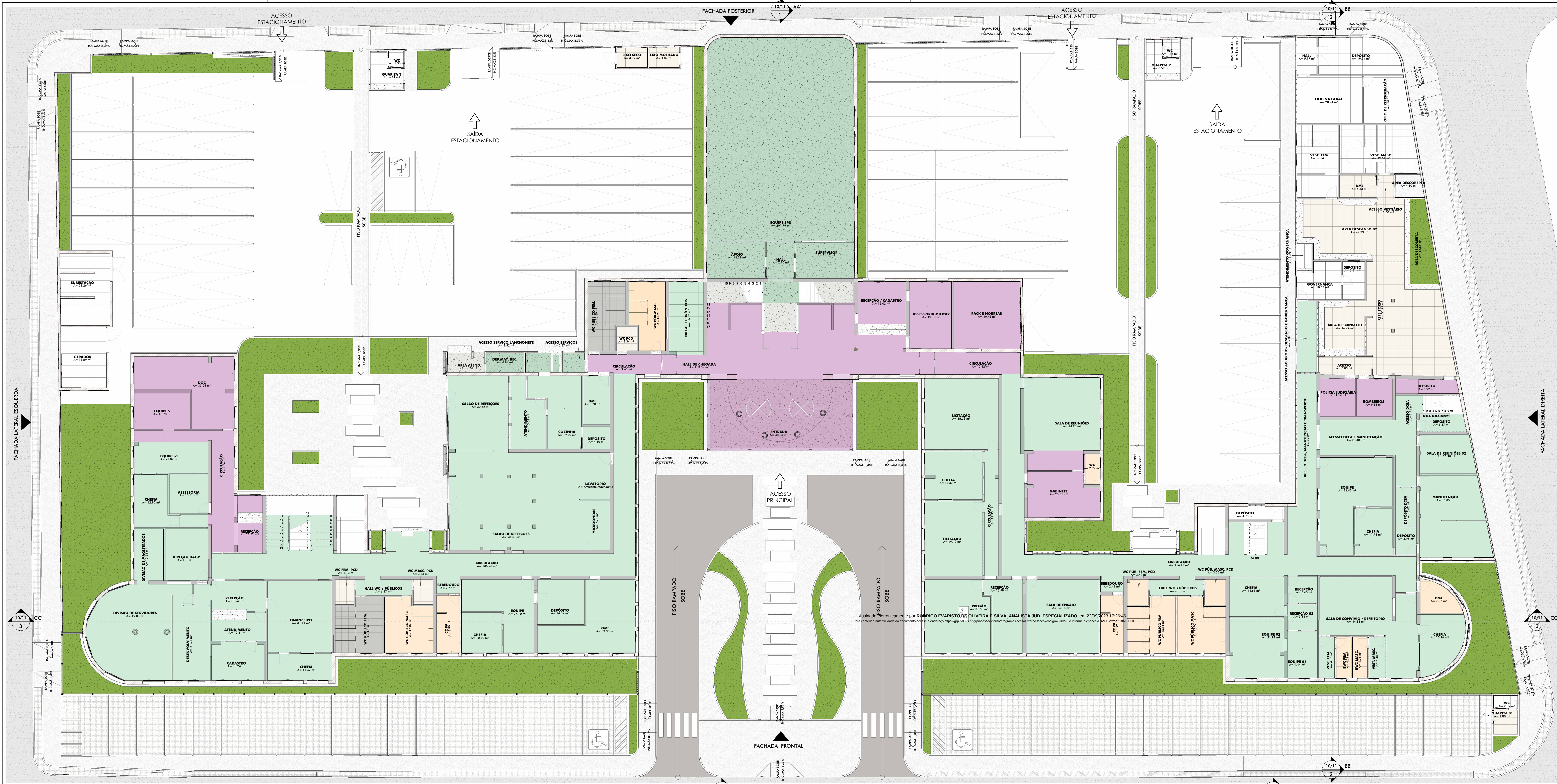
PB DE PAGINAÇÃO DE PISO - TÉRREO ESC:1 : 125
